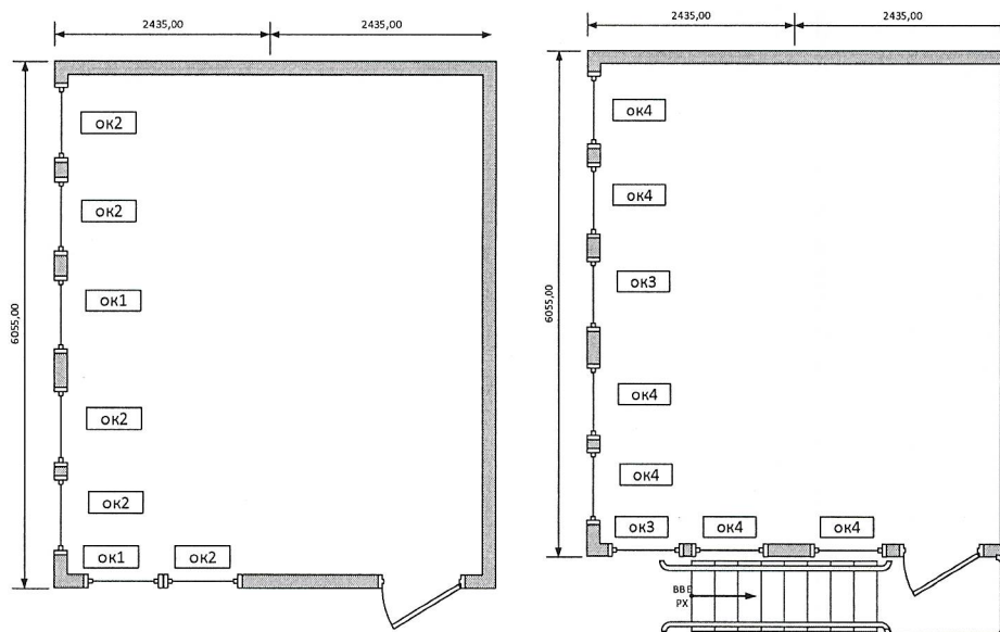
Схема планировки модульного здания
