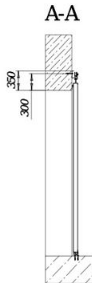
Установка привода
