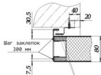
Установка вертикального ДЗ профиля
