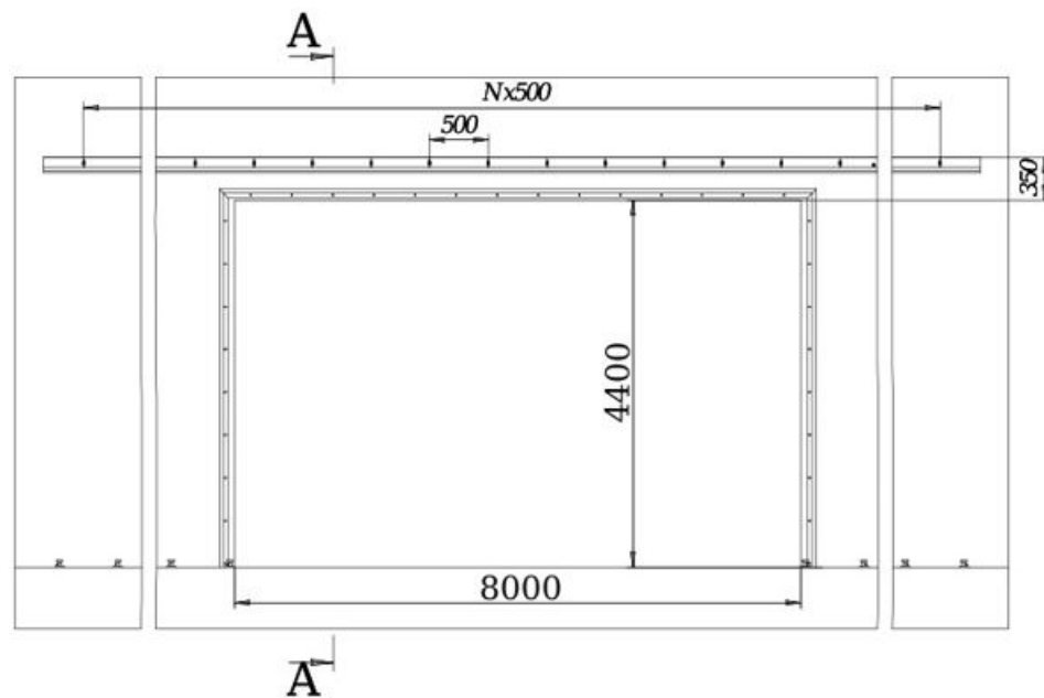
Схема установки балки направляющей (прямой) на проем
