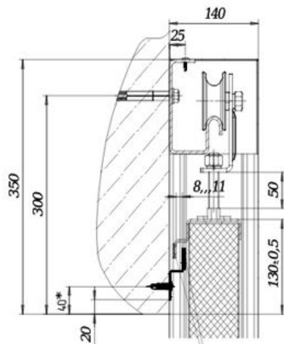
Основные монтажные размеры
