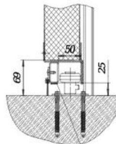
Крепление нижних роликов
