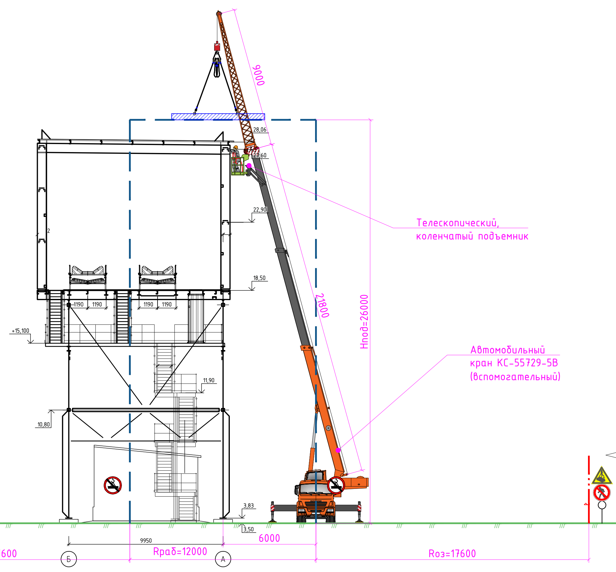
Разрез 2-2 М1:150
