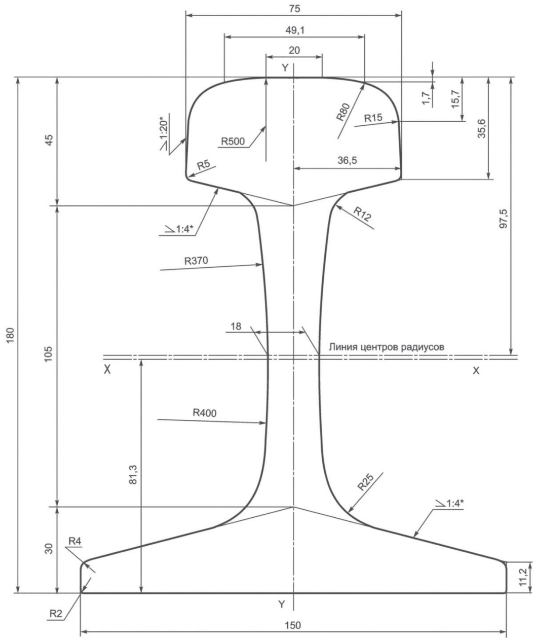
Рисунок 4.2.2.1 Рельс типа Р65
