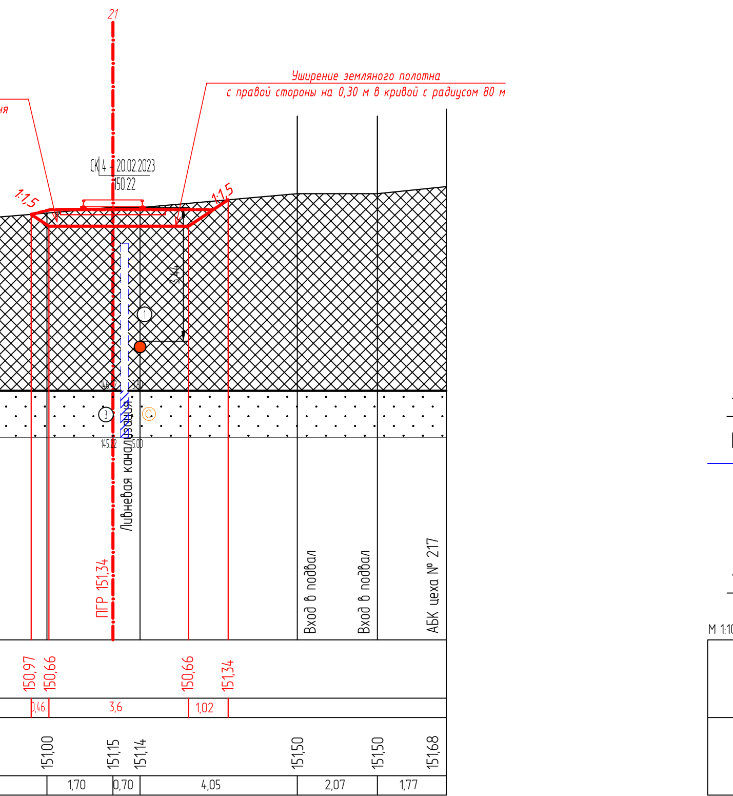
ПК 2+79,27
