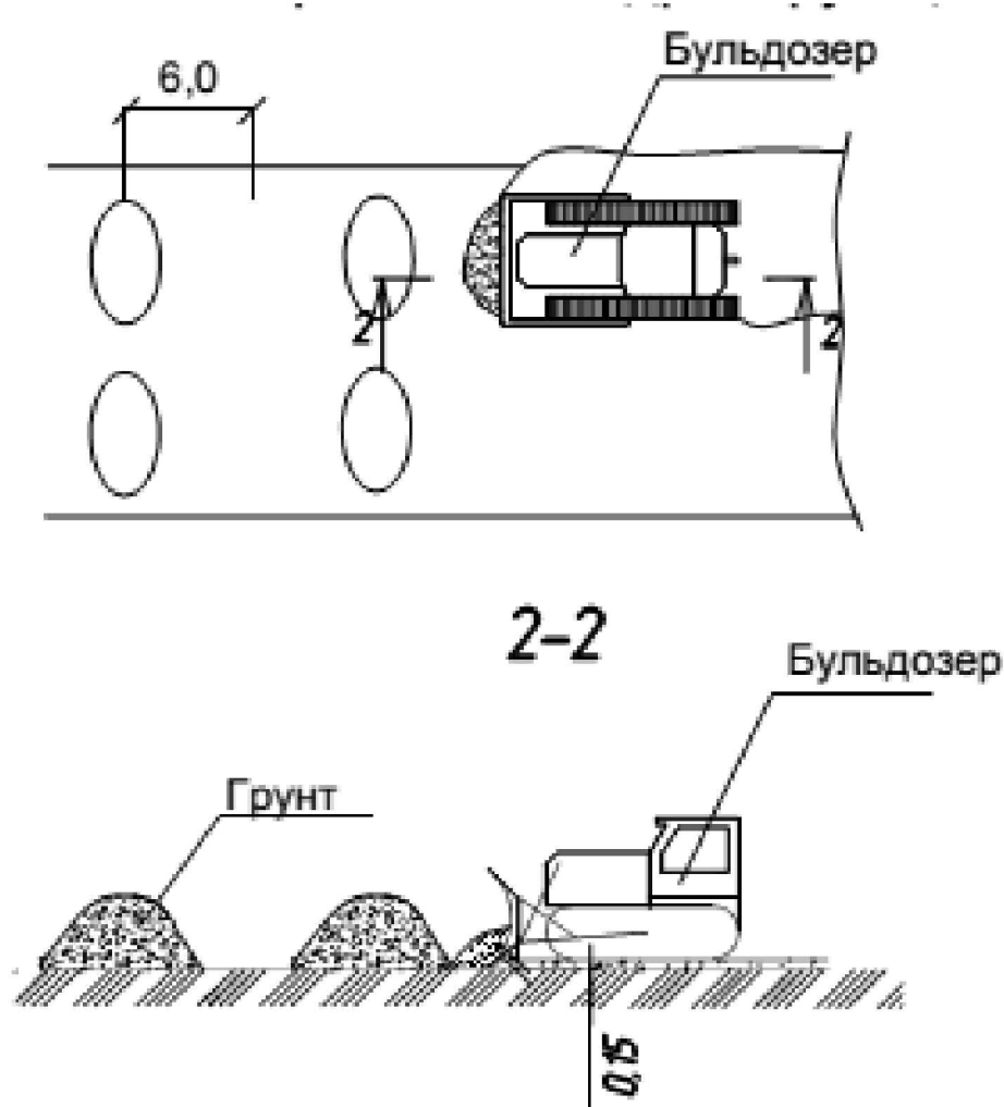
Разравнивание дренирующего грунта бульдозером
