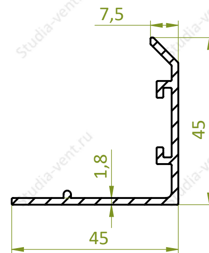
Сечение ламели
