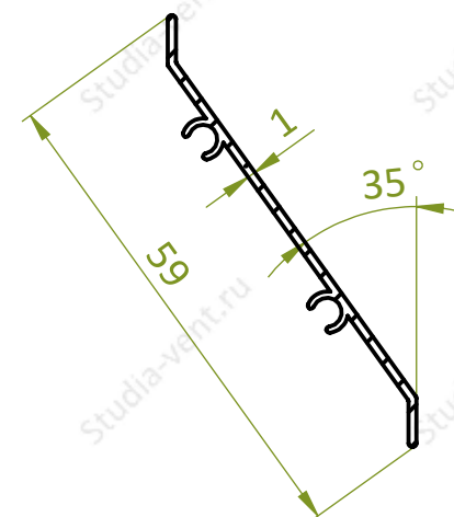
Сечение ламели
