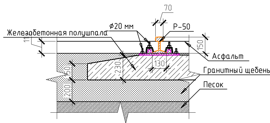
Разрез 1-1
