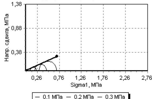
Диаграмма Мора-Кулона
