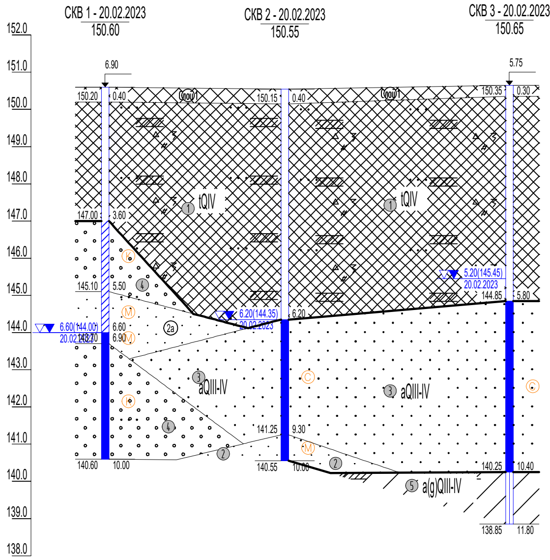
Инженерно-геологический разрез по линии 1-1
