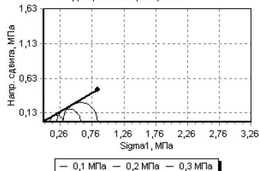
Диаграмма Мора-Кулона
