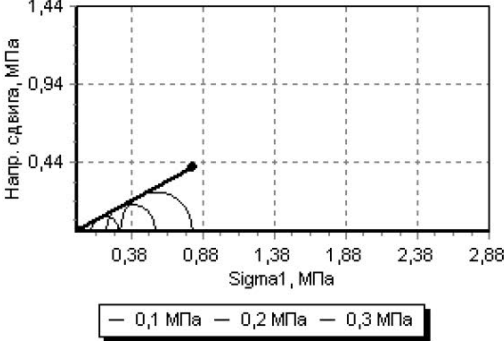
Диаграмма Мора-Кулона
