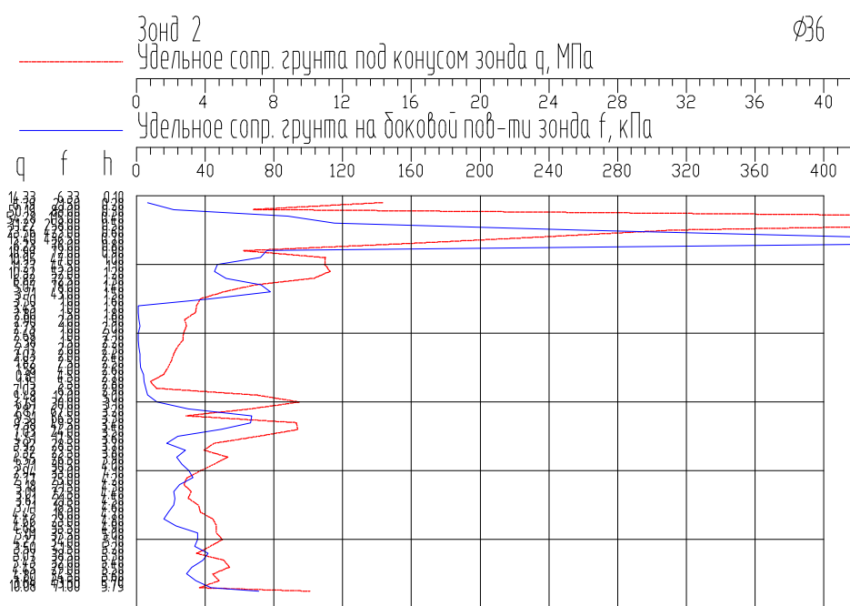
Точка статического зондирования 3
