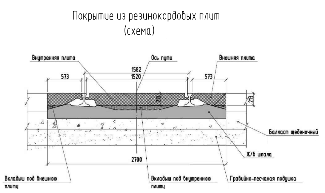
Резинокордовые плиты, проект 2741000 (расход) Общая ширина проездов – 20,00 м
