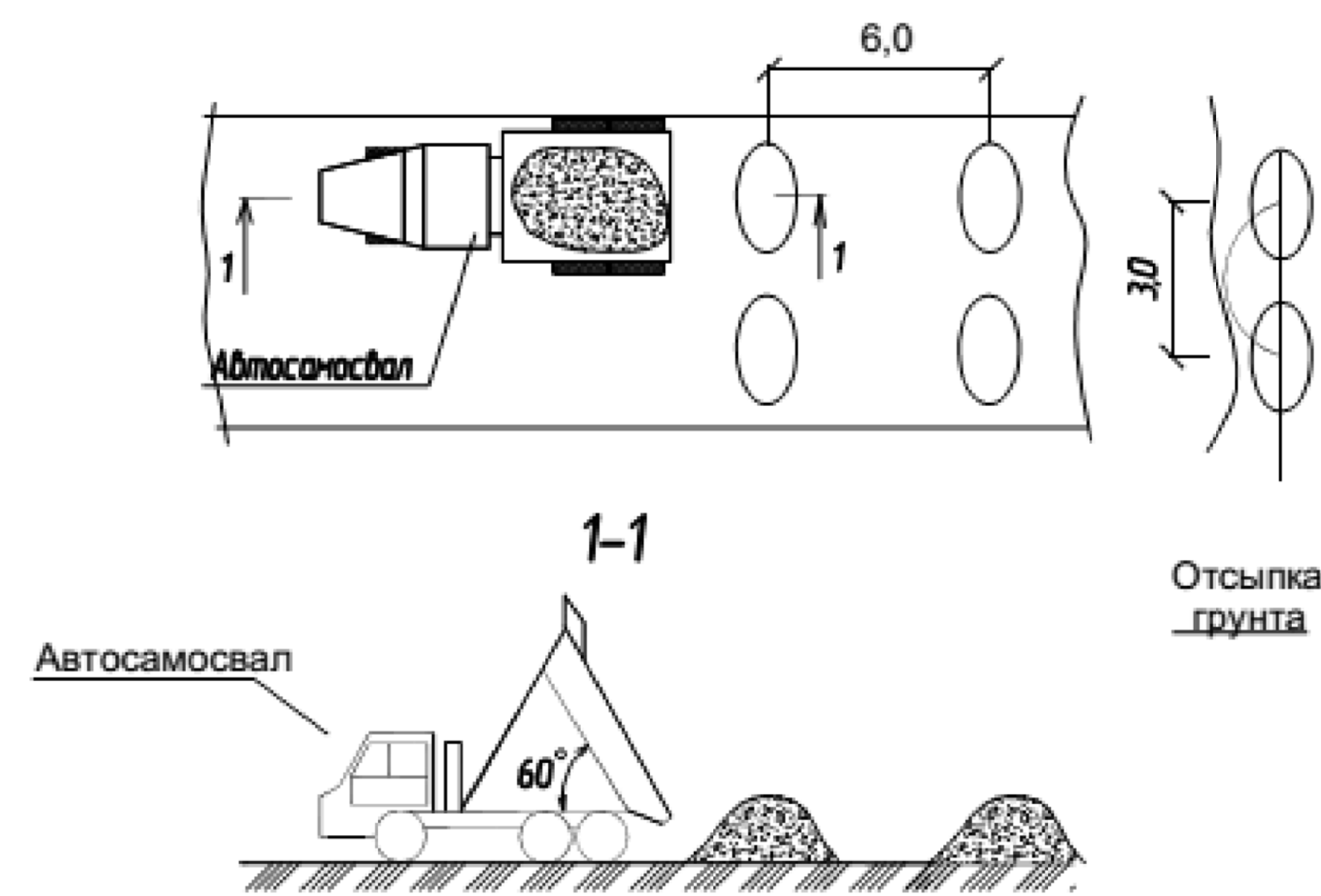
Отсыпканасыпи из дренирующего грунта автосамосвалами
