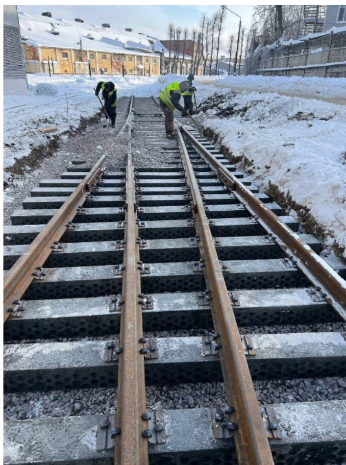
Укладка стрелочного перевода №14 после
