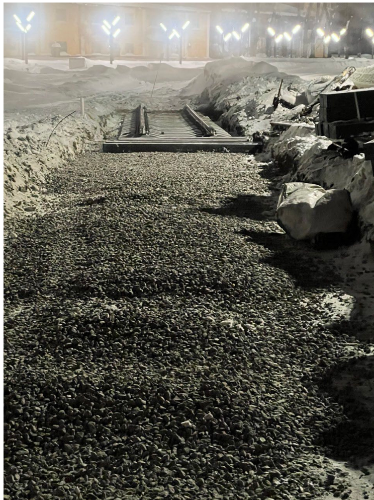
Устройство щебеночного балласта под стрелочный перевод №14 после
