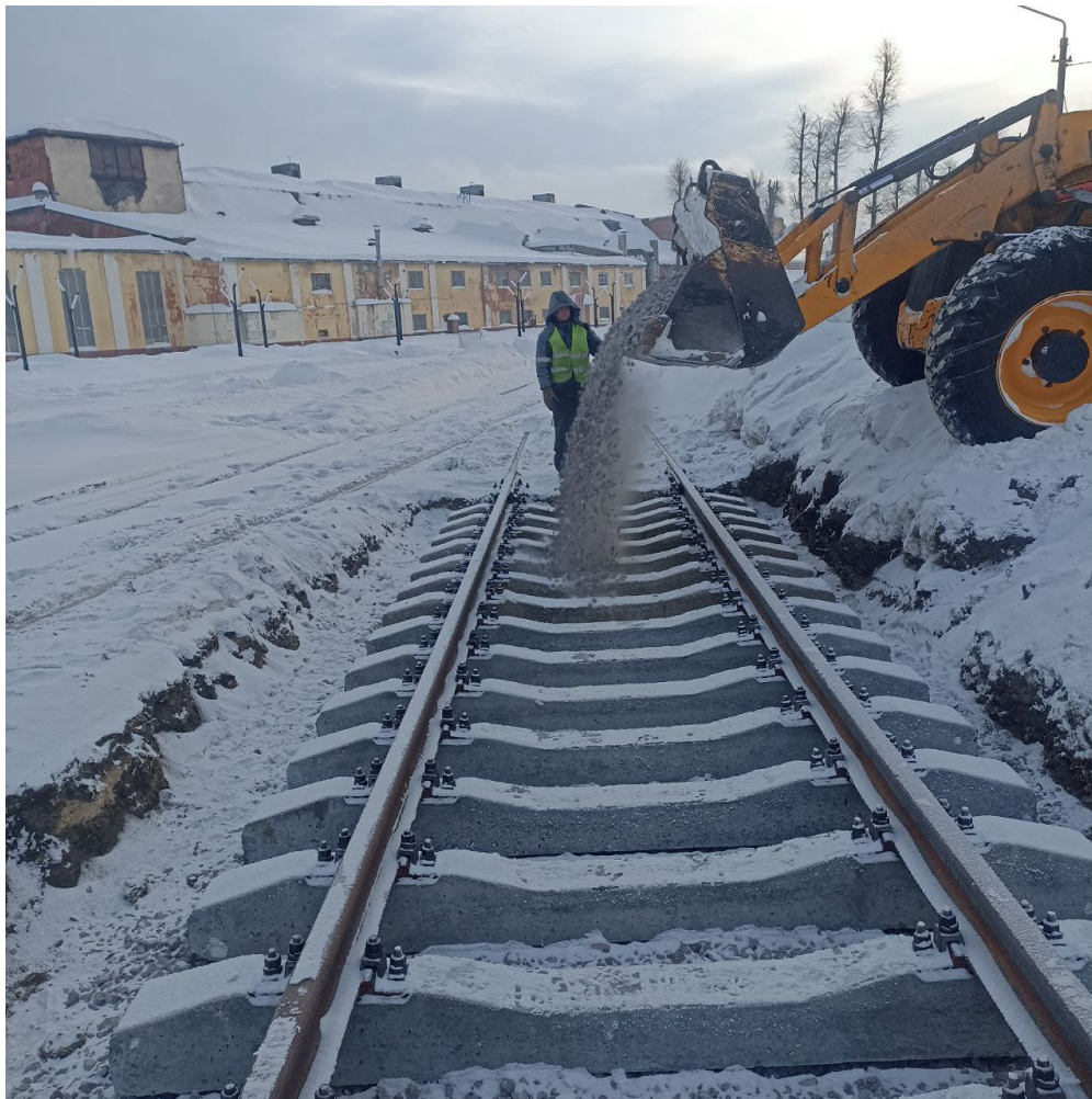
Балластировка, выправка и рихтовка стрелочного перевода №14 до
