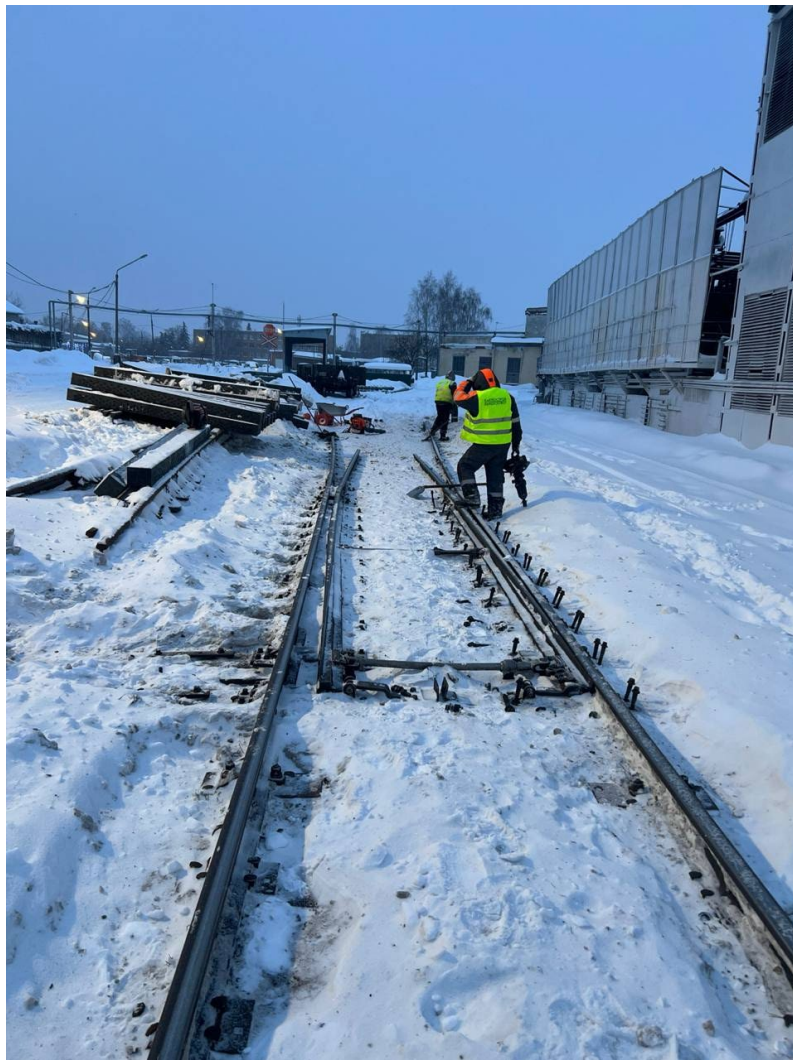
Демонтаж стрелочного перевода №14 до
