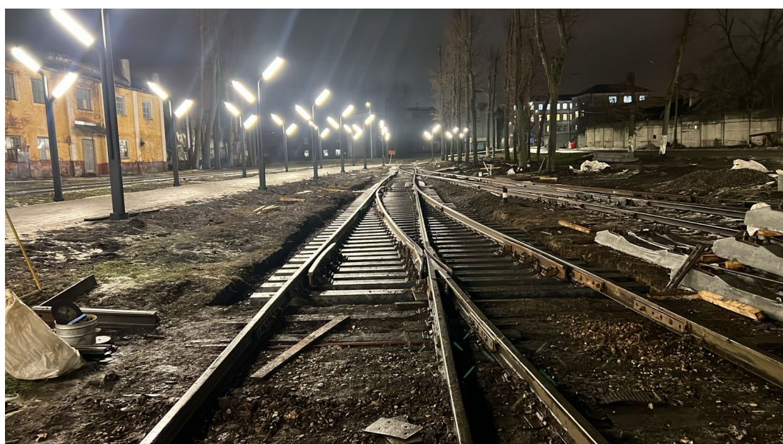
Балластировка, выправка и рихтовка стрелочного перевода №7 после
