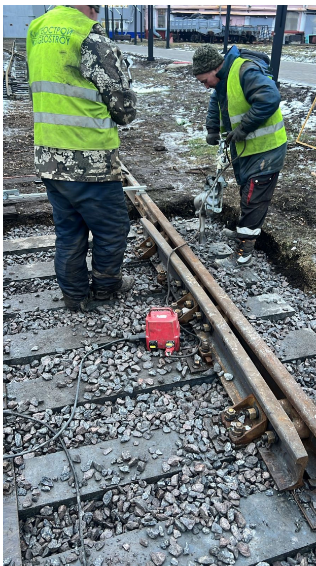
Балластировка, выправка и рихтовка стрелочного перевода №7 до
