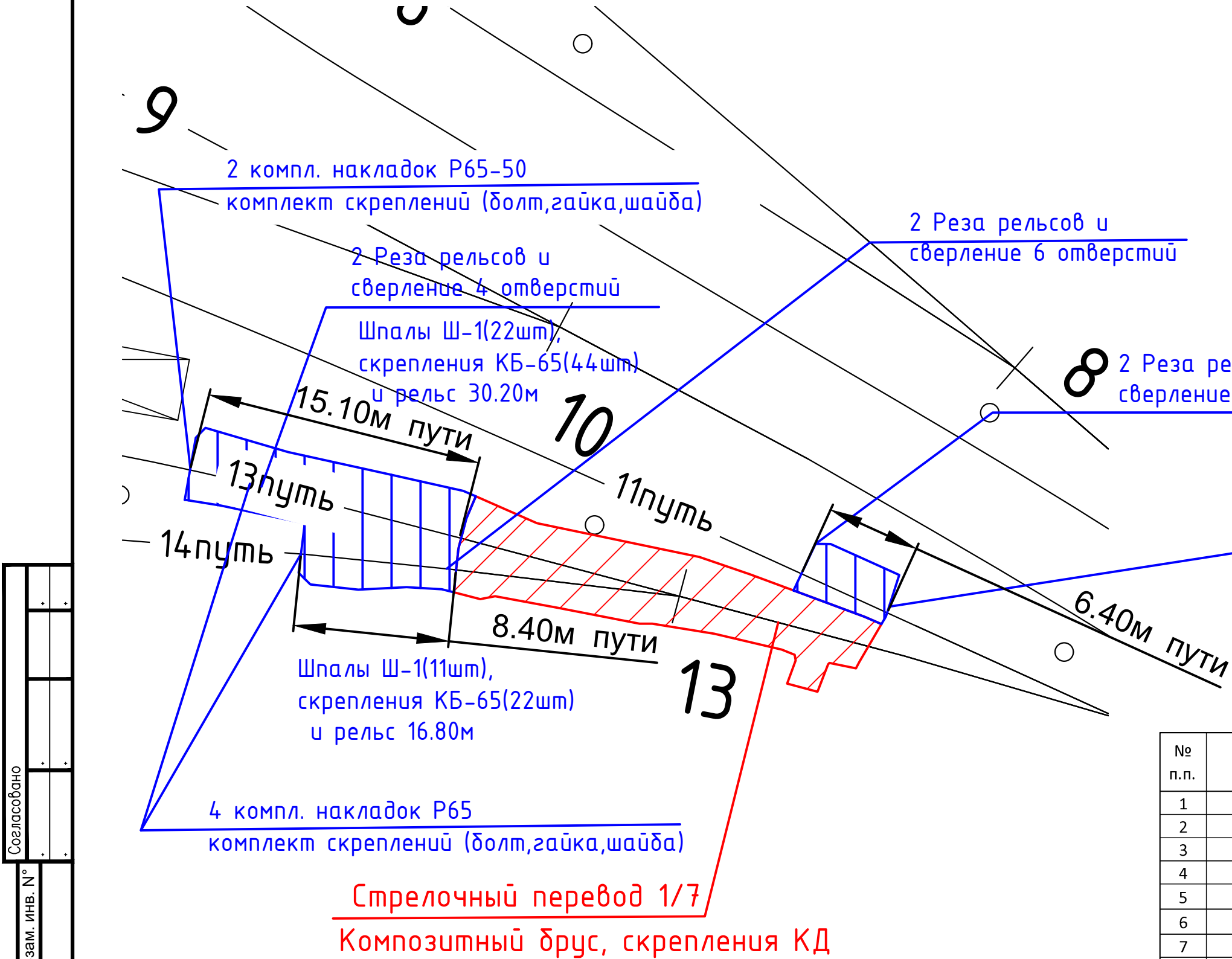
Ведомость объемов работ и материалов по укладке прилежащих жд путей
