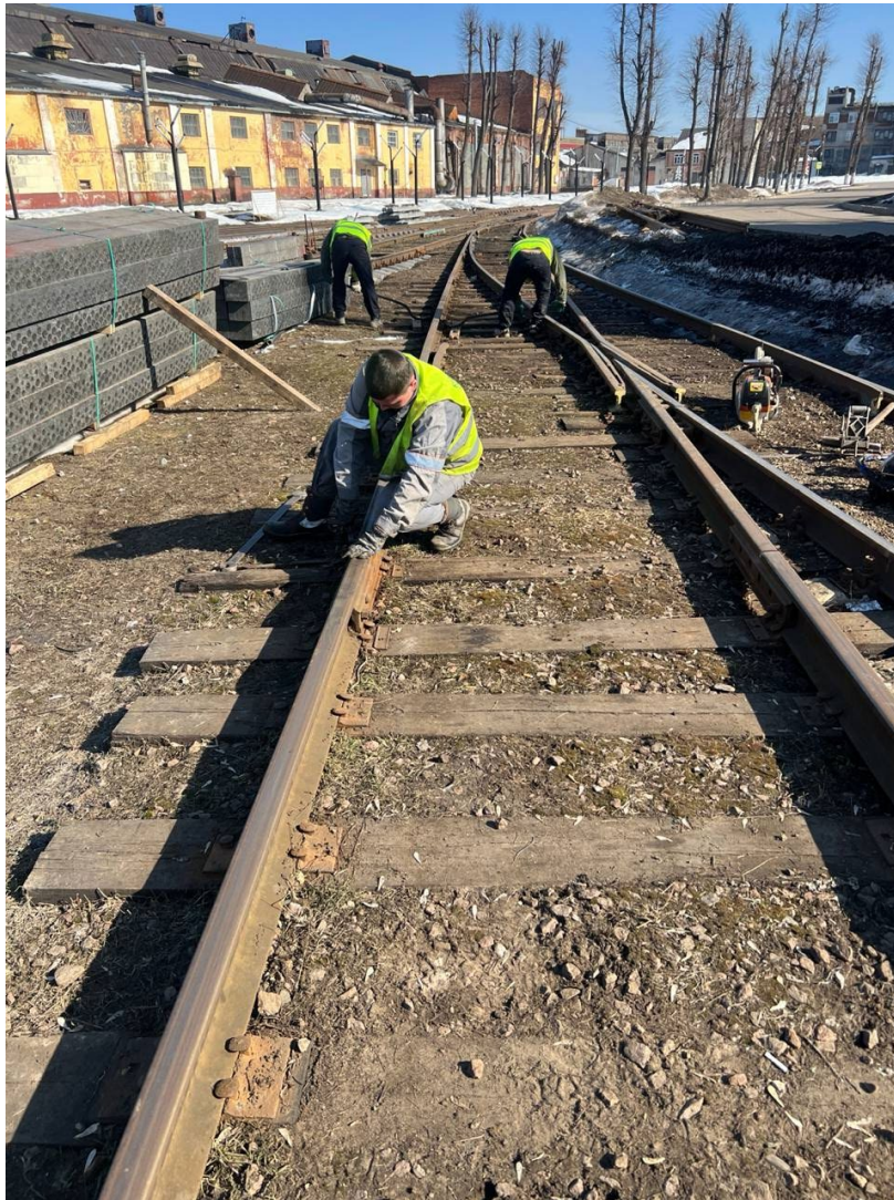
Демонтаж стрелочного перевода №13 до
