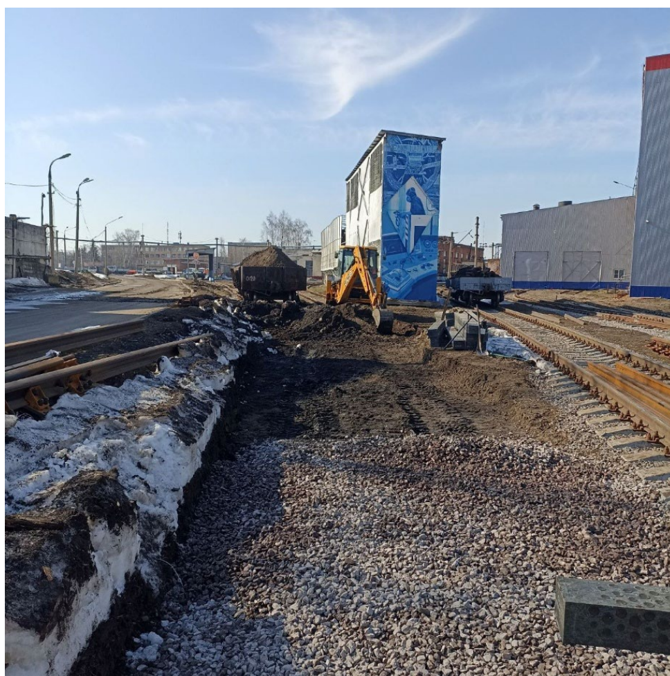
Выемка загрязненного балласта под стрелочный перевод №13 после
