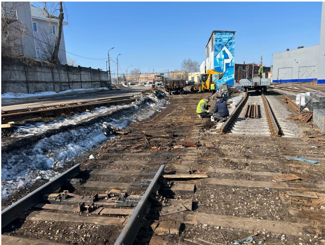
Демонтаж стрелочного перевода №13 после
