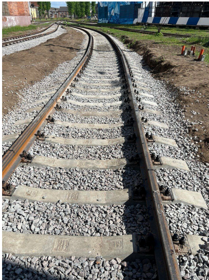
Балластировка, выправка и рихтовка путей №9 и №10 после
