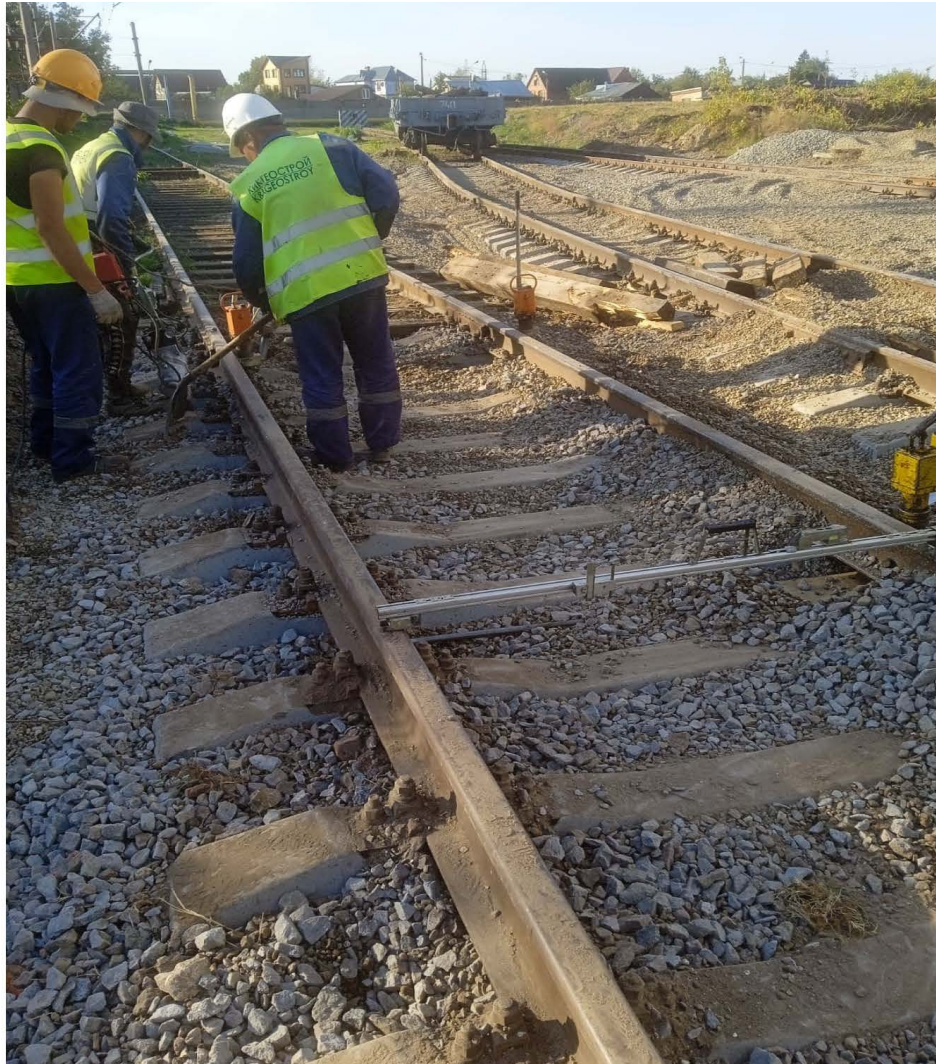
Балластировка стрелочного перевода №12 на жд. пути №11 после
