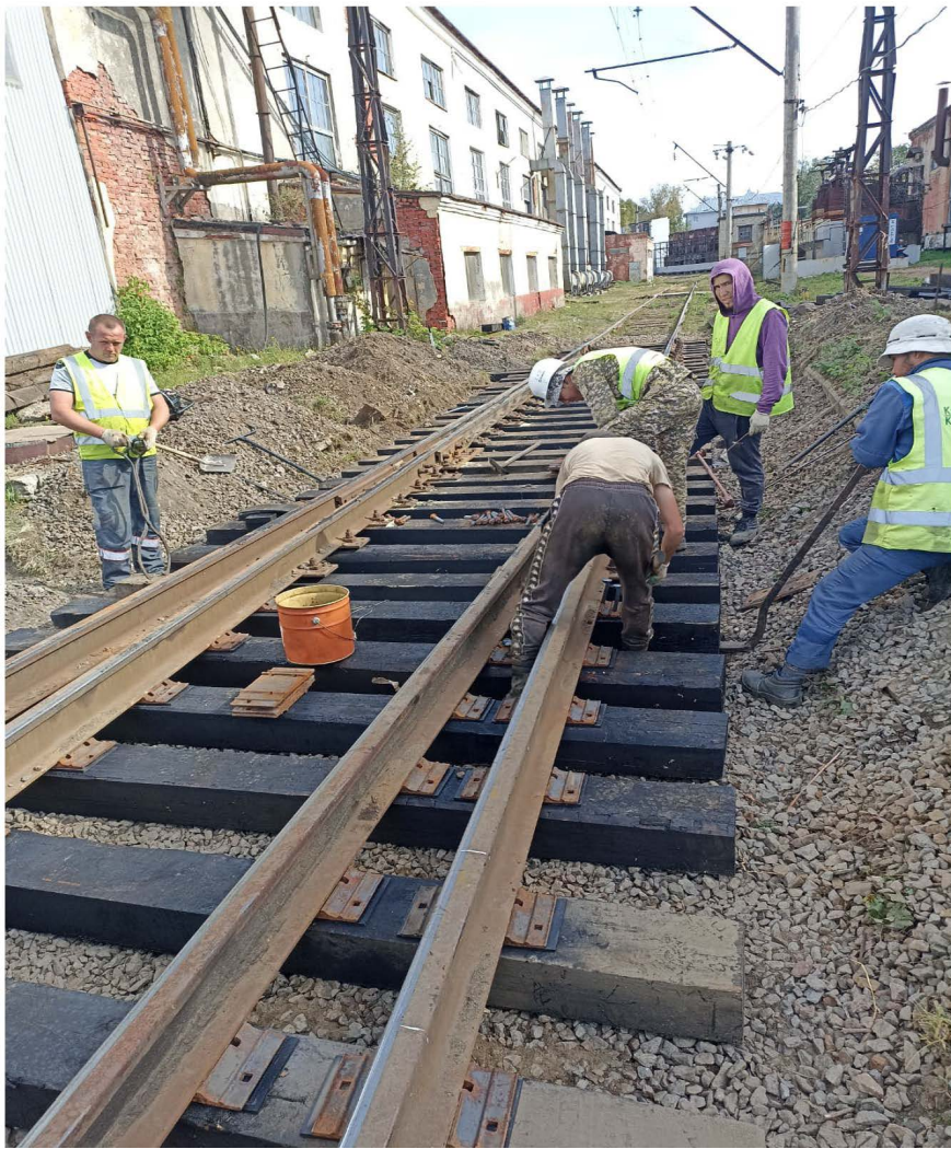
Внесение дополнительного щебня стрелочного перевода №12 на жд. пути №11 после
