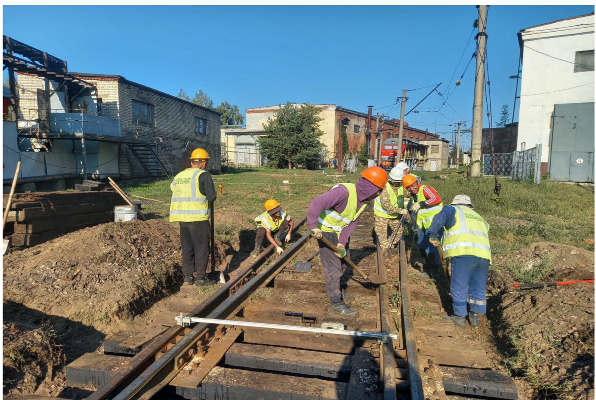
Внесение дополнительного щебня в основание стрелочного перевода №126 на жд. пути №11 до
