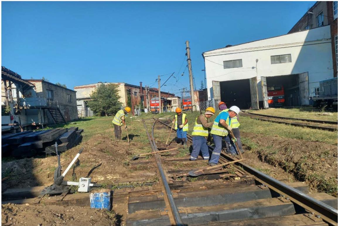
Очистка стрелочного перевода №126 на жд. пути №11 до
