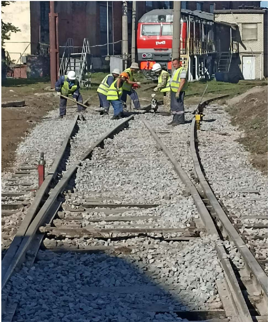
Балластировка стрелочного перевода №126 на жд. пути №11 после
