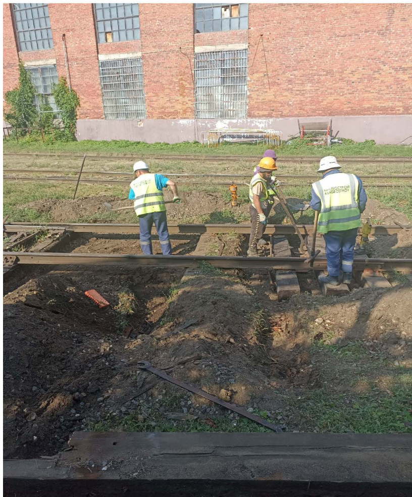
Очистка стрелочного перевода №126 на жд. пути №11 после
