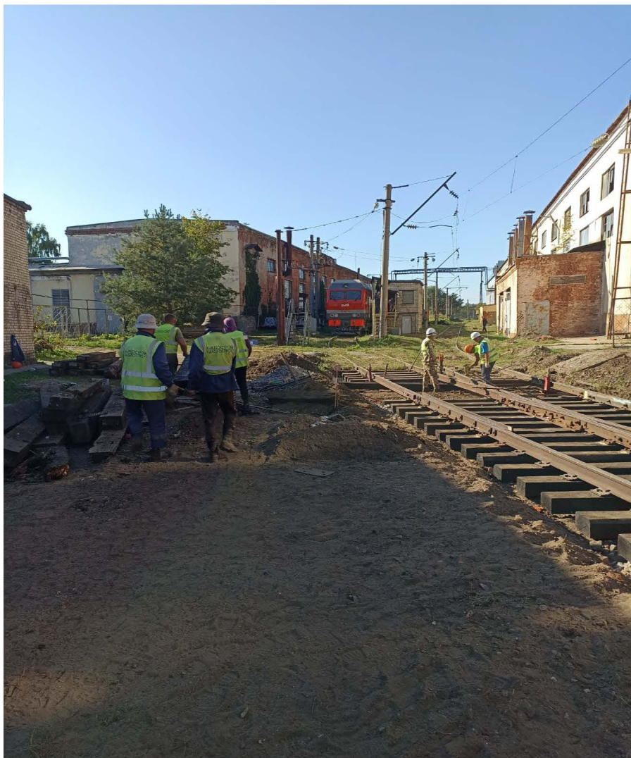
Ремонт стрелочного перевода №126 на жд. пути №11 после
