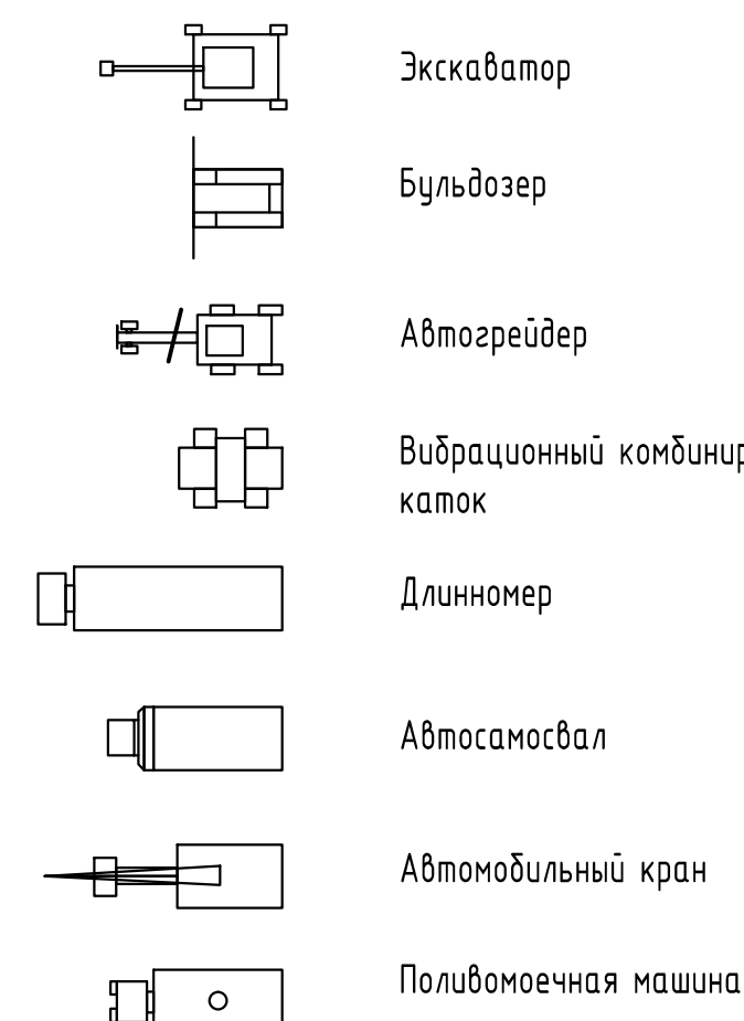
Условные обозначения строительной техники
