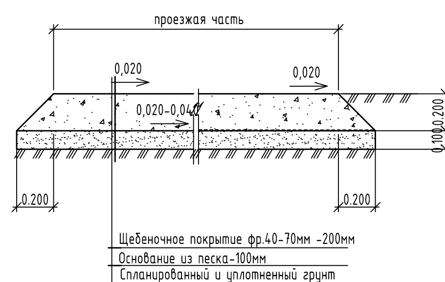
Конструкция временного автопроезда
