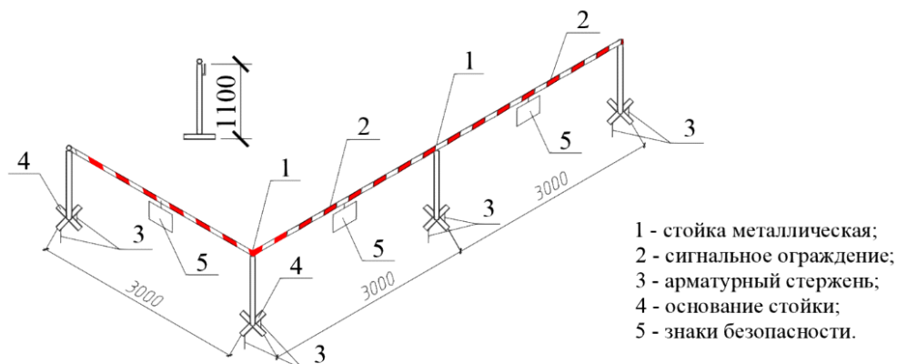
Схема устройства ограждения опасных зон
