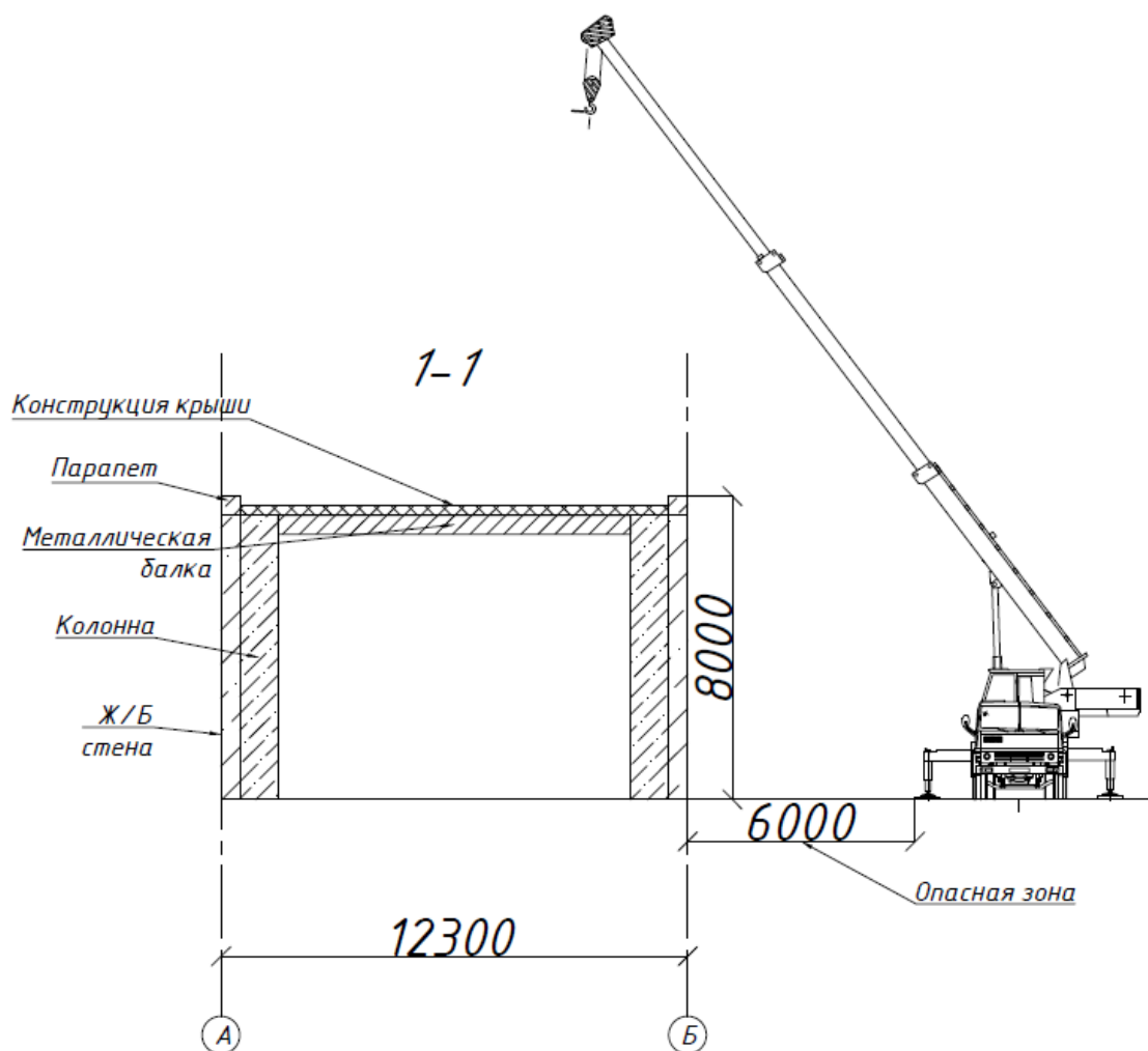
Схема демонтажа конструкций при помощи крана
