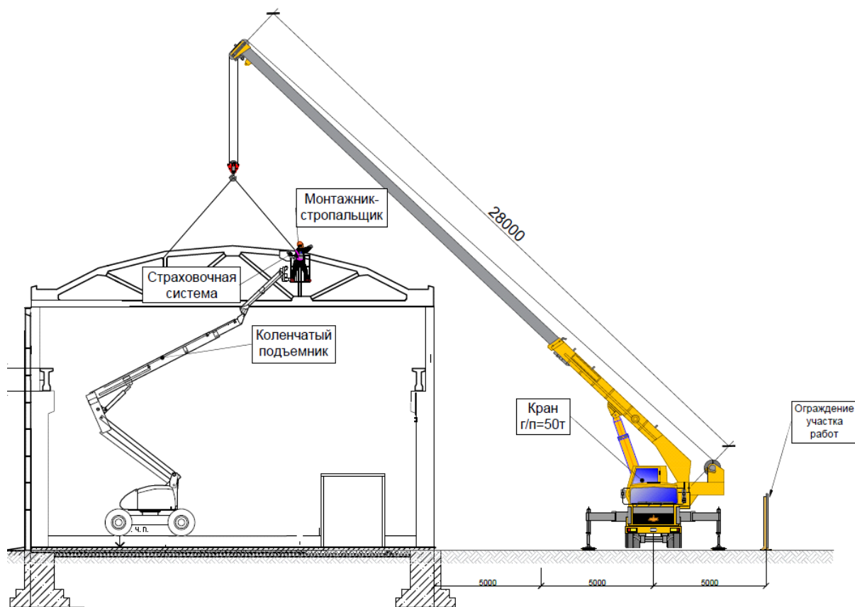
Схема выполнения строповки с подъемника снаружи корпуса
