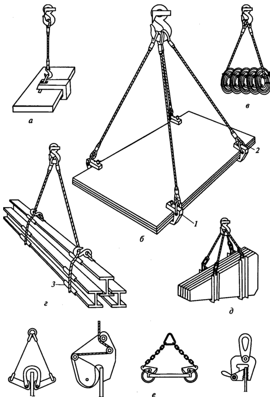
Схема строповки грузов
