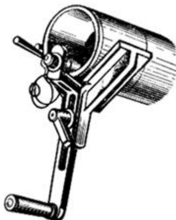
Рис.1. Устройство для торцовки и снятия фасок
