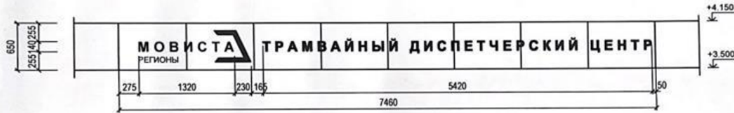
Схема вывески М1:50
