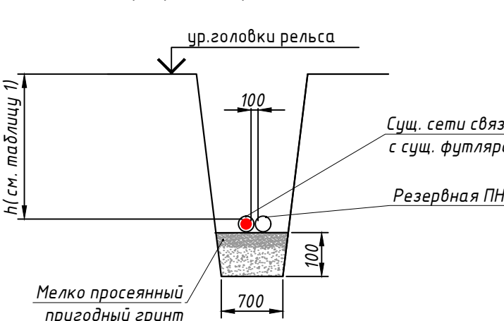
Разрез 2-2 Профиль траншеи
