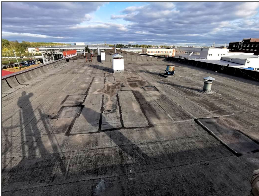
Фото 7. Общий вид кровли здания в осях А-Гх5-9. Отмечены участки периодических ремонтов гидроизоляционного ковра, участки застаивания атмосферных вод
