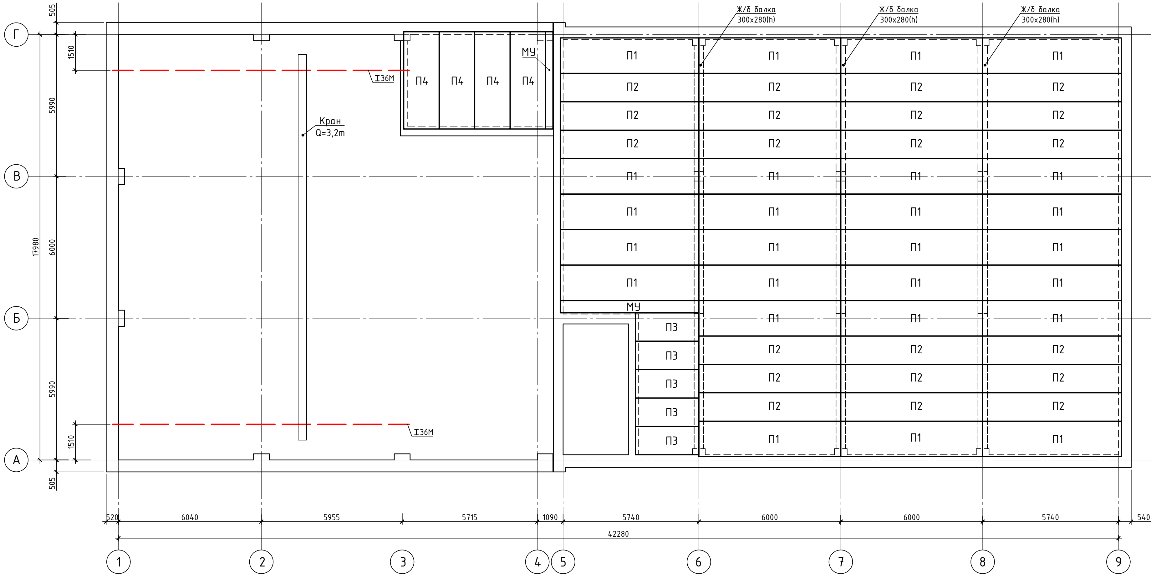
Схема несущих конструкций перекрытия над 1-ым этажом
