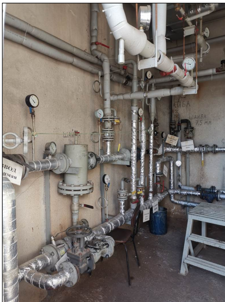
Фото 12. Общий вид оборудования теплового пункта
