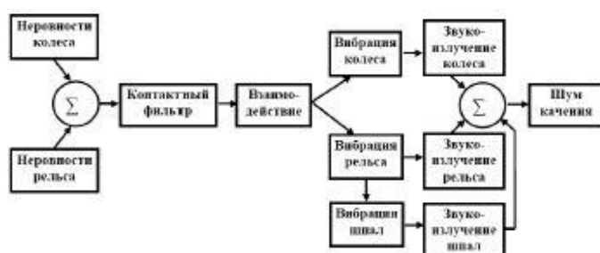
Рис. 4. Графический вид модели процесса образования шума качения
