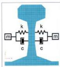
Схематичное изображение рельсового абсорбера
