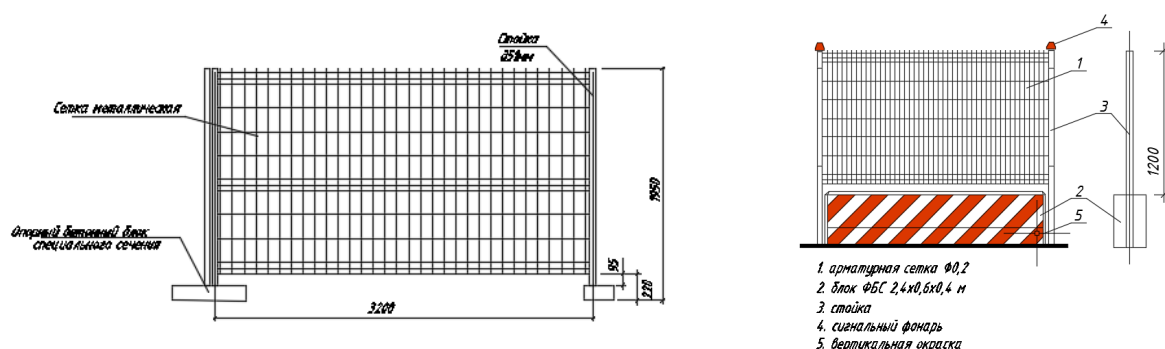
Рисунок 1 – Ограждения типа 1АН и 2АН
