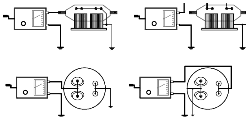
Рис 6.1. Схема измерения сопротивления изоляции трансформаторов
