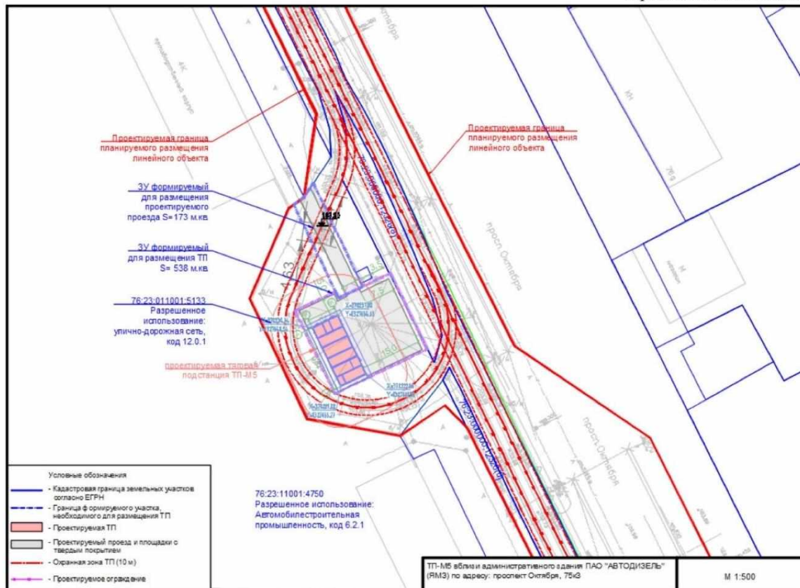
Рисунок 1. Обзорная схема расположения проектируемой ТП-М5
