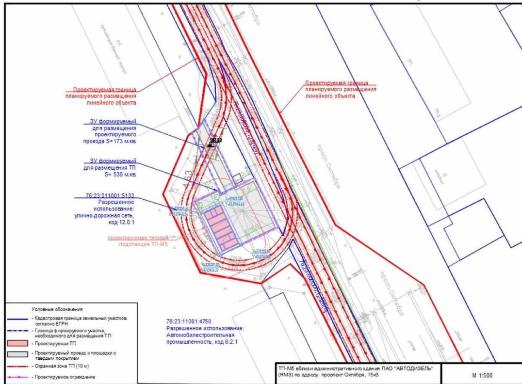
Рисунок 1. Обзорная схема расположения проектируемой ТП-М5
