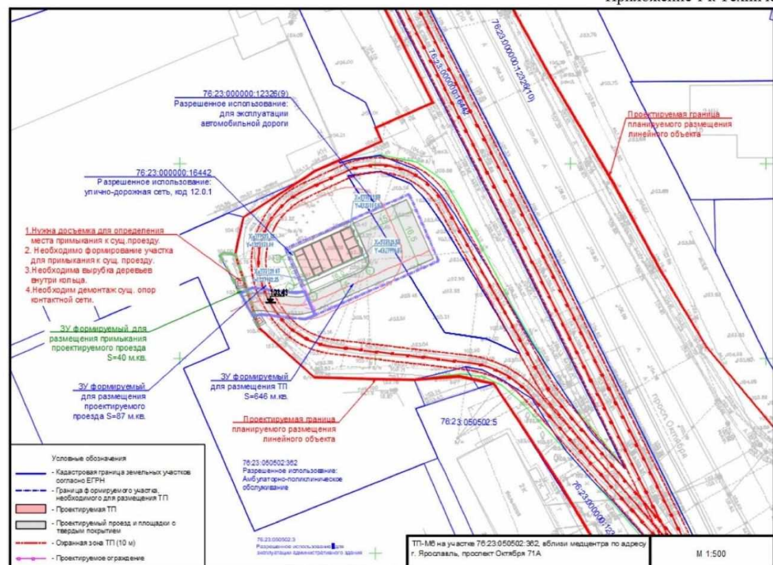
Рисунок 2. Обзорная схема расположения проектируемой ТП-М6
