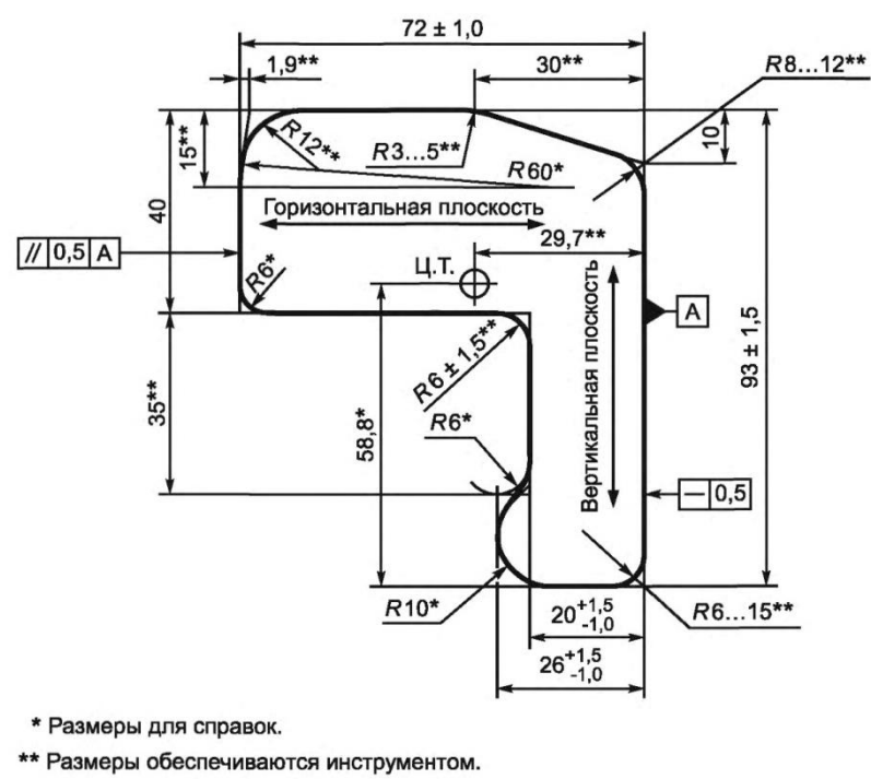
Рисунок 4.3.9.1 Размеры поперечного сечения уголков типа СП850
