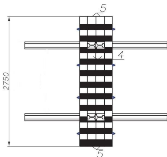
Рисунок 4.3.10.1 Железнодорожный тупиковый упор ТУ 5264-001-83875090-2016
