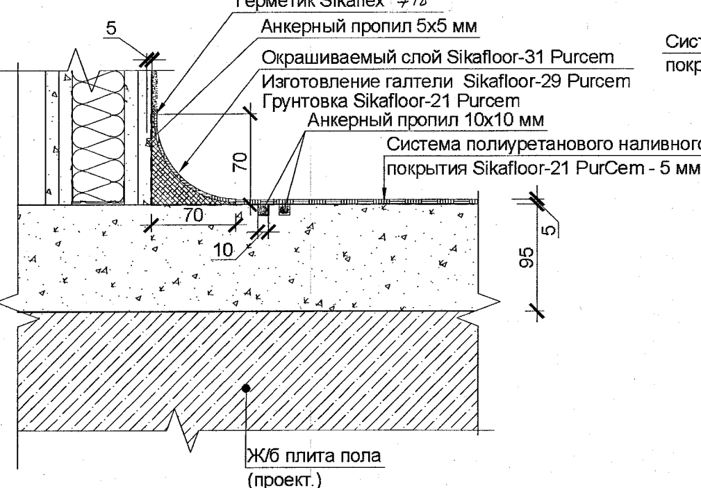
Узел примыкания покрытия пола по системе Sika к каркасной перегородке (для полов типа 2.1) М 1:10
