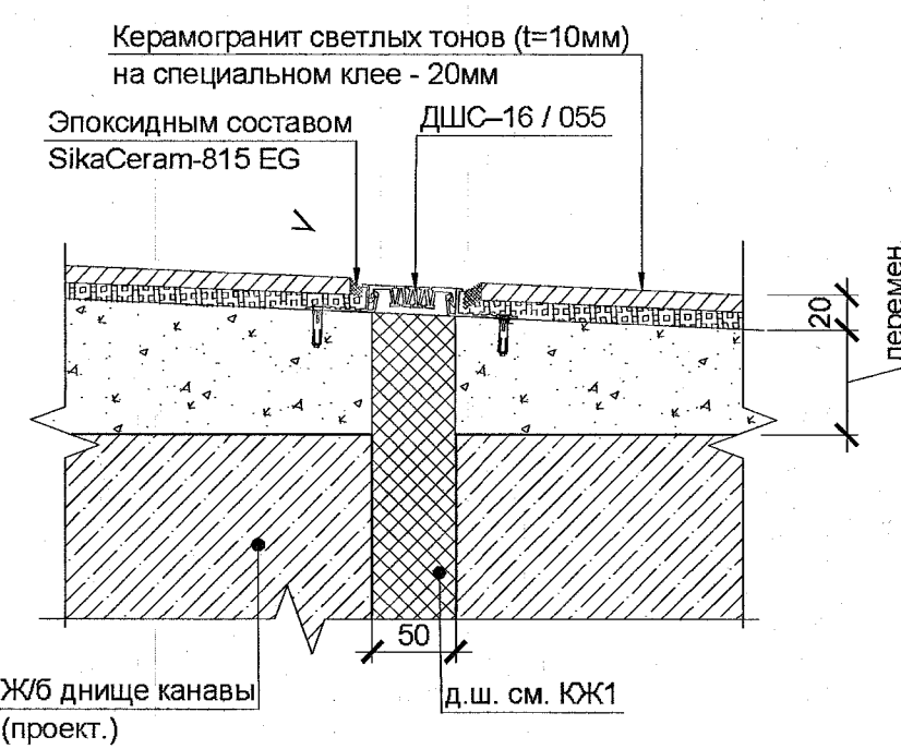
Узел примыкания покрытия пола к деформационным швам (для полов типа 4) М 1:10
