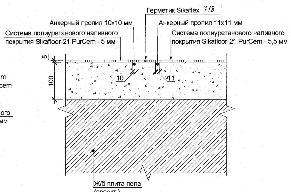
Узел примыкания покрытия пола по системе Sika к ж.д. путям (для полов типа 2.2) М 1:10
