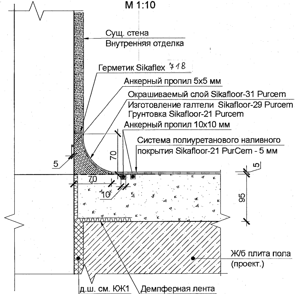
Узел примыкания покрытия пола по системе Sika к кирпичным перегородке (для полов типа 2.1) М 1:10
