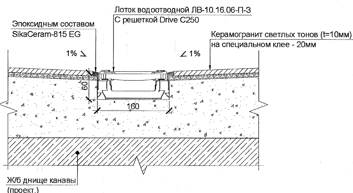
Узел примыкания покрытие пола к лотку в смотровой канаве (для полов типа 4) М 1:10
