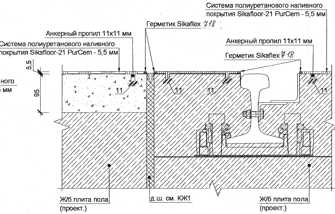
Узел примыкания покрытия пола по системе Sika к ж.д. путям (для полов типа 2.2) М 1:10
