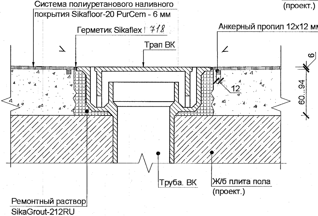
Узел примыкания покрытие пола к лотку в смотровой канаве (для полов типа 4) М 1:10
