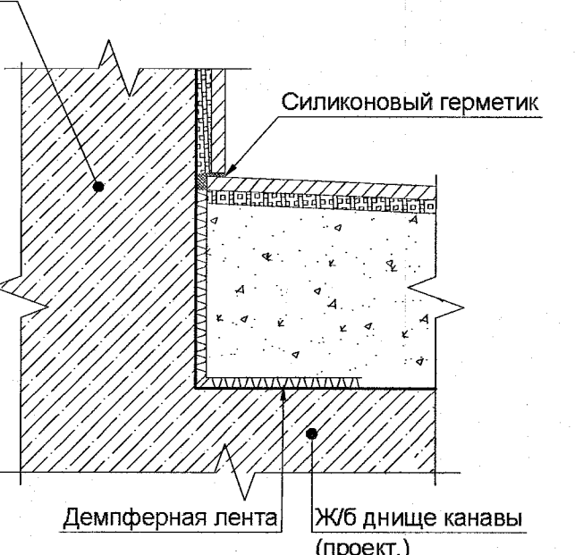
Узел примыкания покрытие пола к стенам канавы (для полов типа 4) М 1:10
