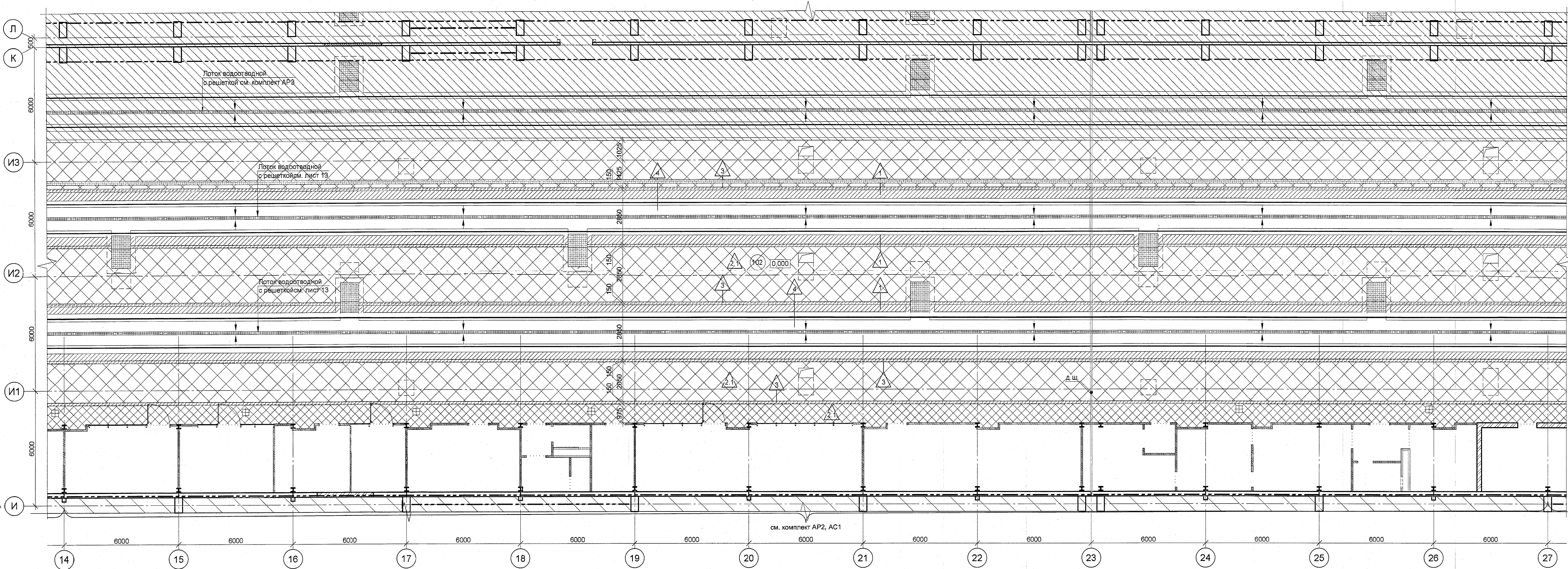
Схема полов на отм. 0,000 между осями 14-27 и И-И3 М 1:100
