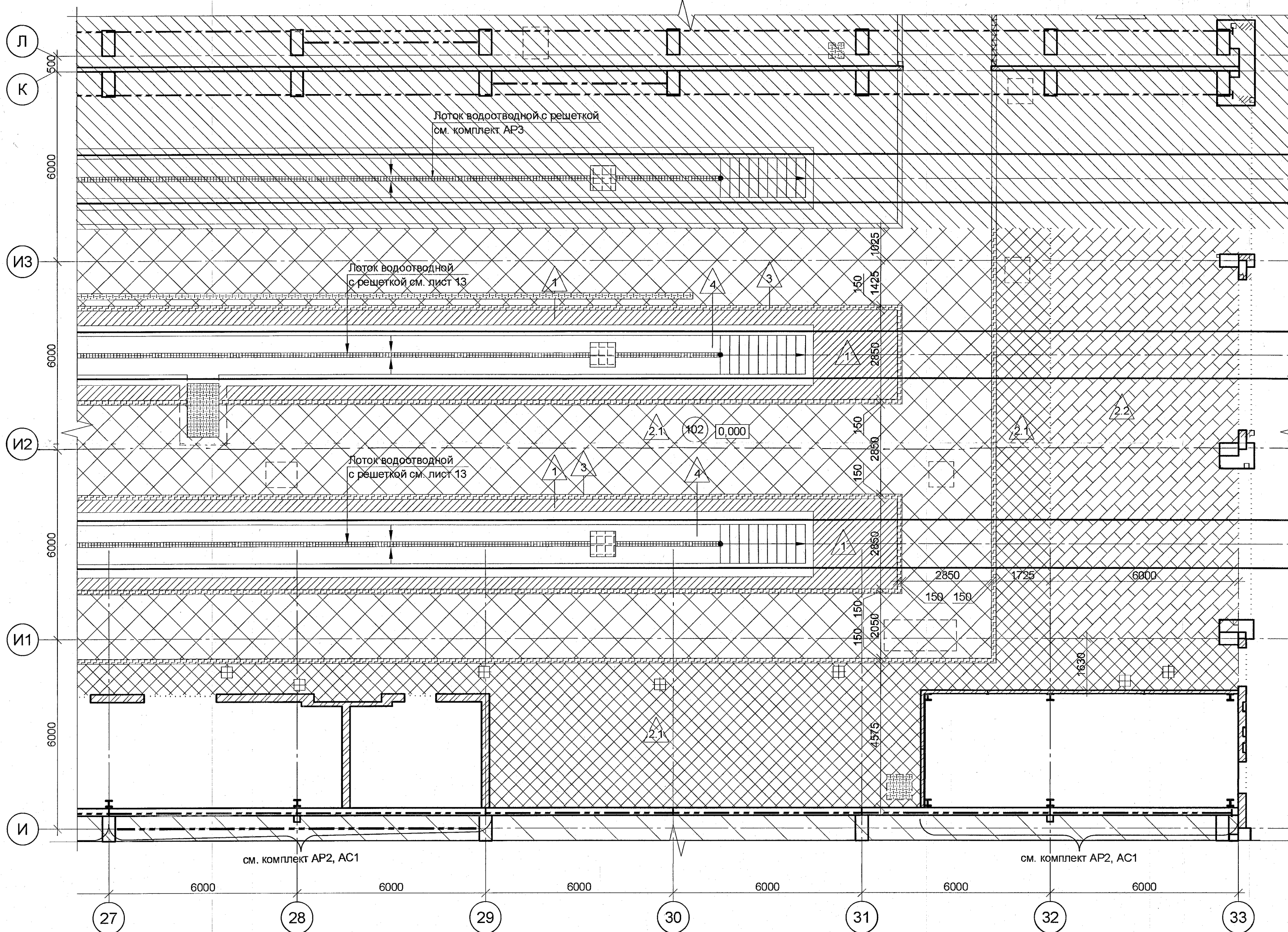
Схема полов на отм. 0,000 между осями 27-33 и И-ИЗ М 1:100
