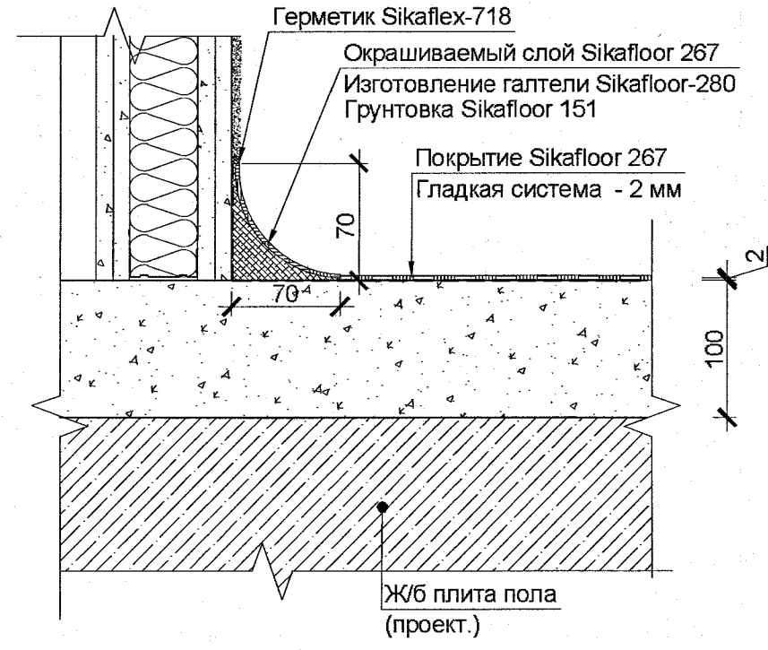
Узел примыкания покрытия пола к каркасным перегородкам (для полов типа 8) М 1:10
