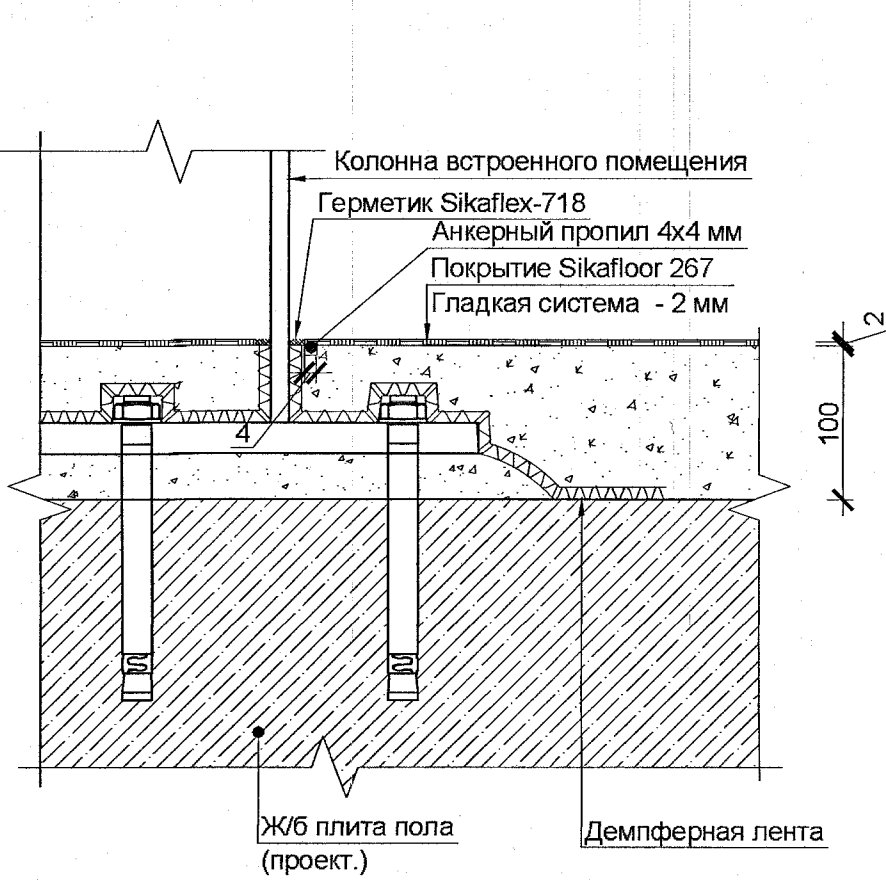
Узел примыкания покрытия пола к каркасным перегородкам (для полов типа 9) М 1:10
