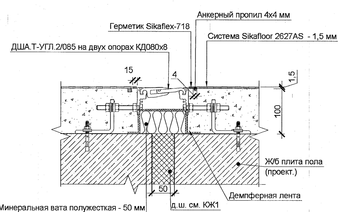
Узел примыкания покрытия пола к деформационным швам (для полов типа 9) М 1:10
