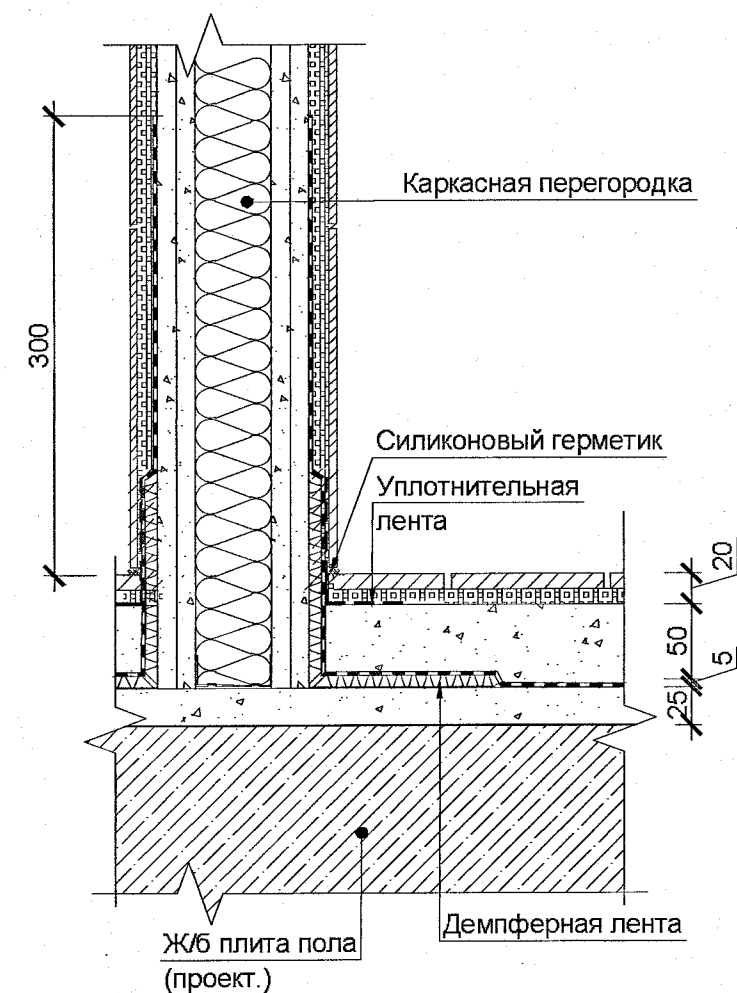
Узел примыкания покрытия пола к существующим стенам (для полов типа 7) М 1:10
