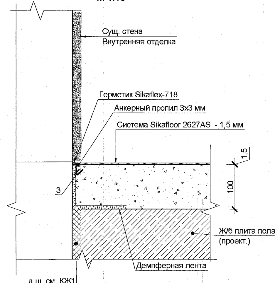
Узел примыкания покрытия пола к существующим стенам (для полов типа 9) М 1:10
