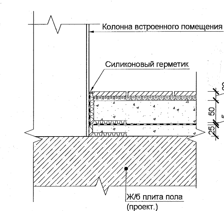
Узел примыкания покрытия пола к проектируемым колоннам (для полов типа 7) М 1:10
