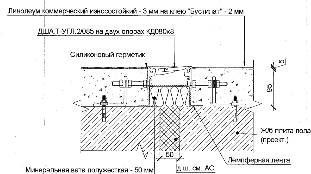
Узел примыкания покрытия пола к деформационным швам (для полов типа 10) М 1:10
