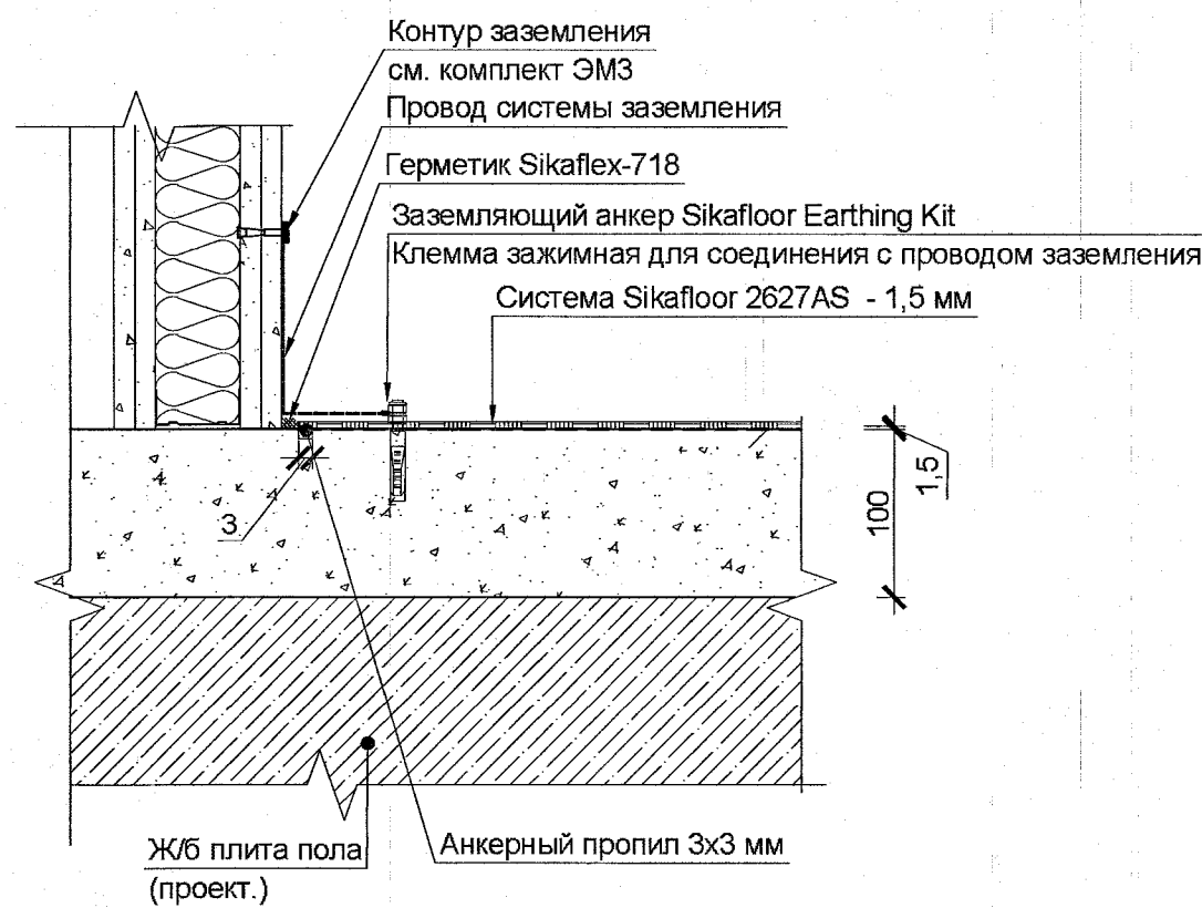
Узел примыкания покрытия пола к существующим стенам (для полов типа 9) М 1:10
