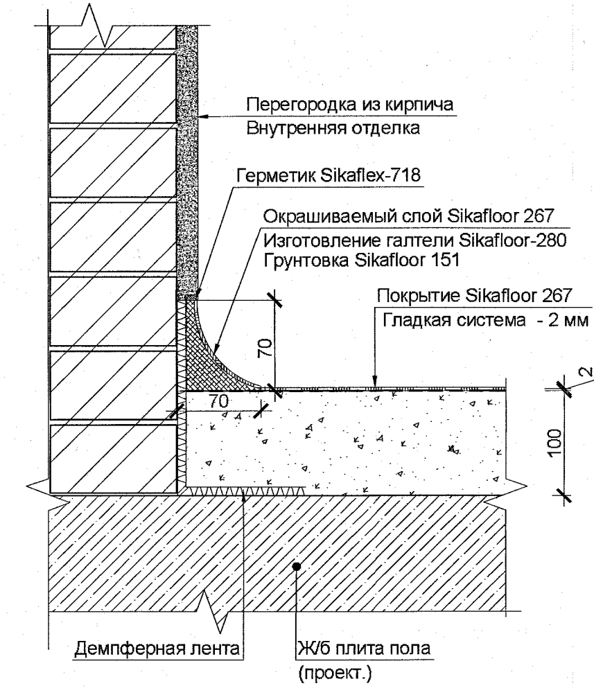
Узел примыкания покрытия пола к существующим стенам (для полов типа 8) М 1:10
