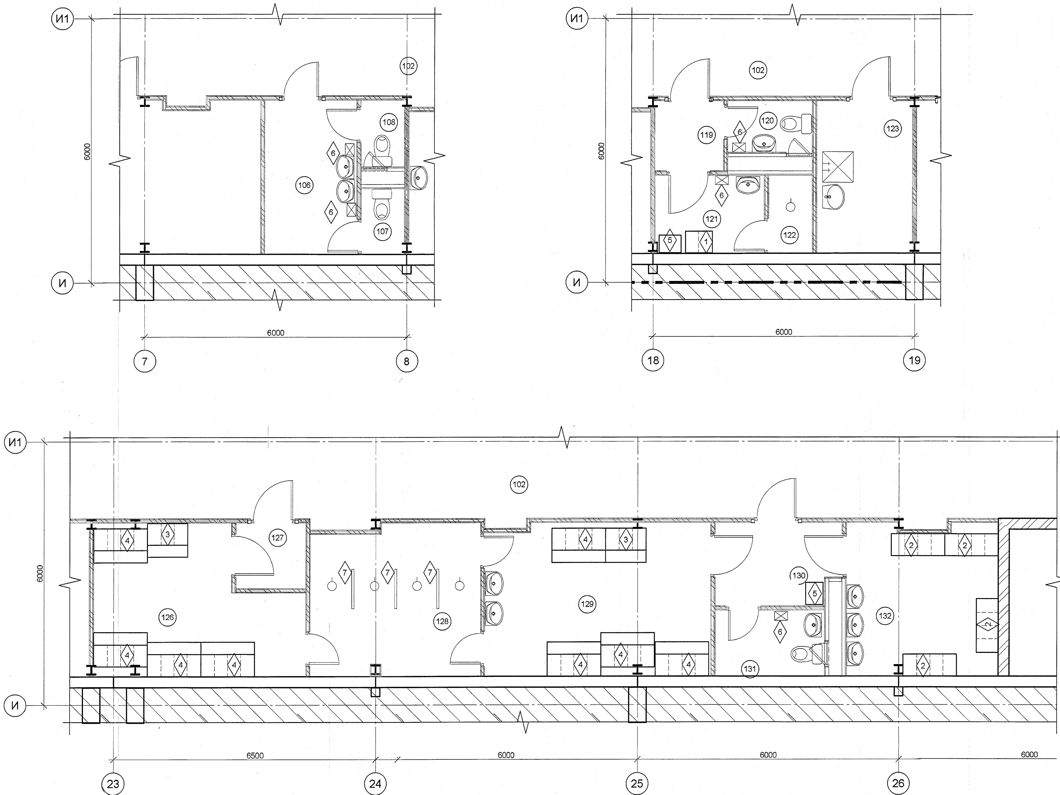
План с расстановкой оборудования бытовых помещений на отм. 0,000 между осями 7-8 и И-И1, 18-19 и И-И1, 23-26 и И-И1 М 1:50
