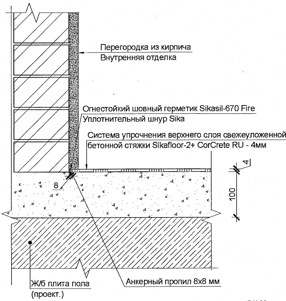
Узел примыкания покрытия пола по системе Sika к существующим стенам (для полов типа 5) М 1:10
