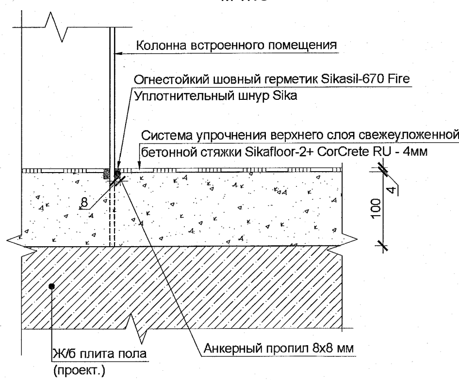
Узел примыкания покрытия пола по системе Sika к проектируемым колоннам (для полов типа 5) М 1:10
