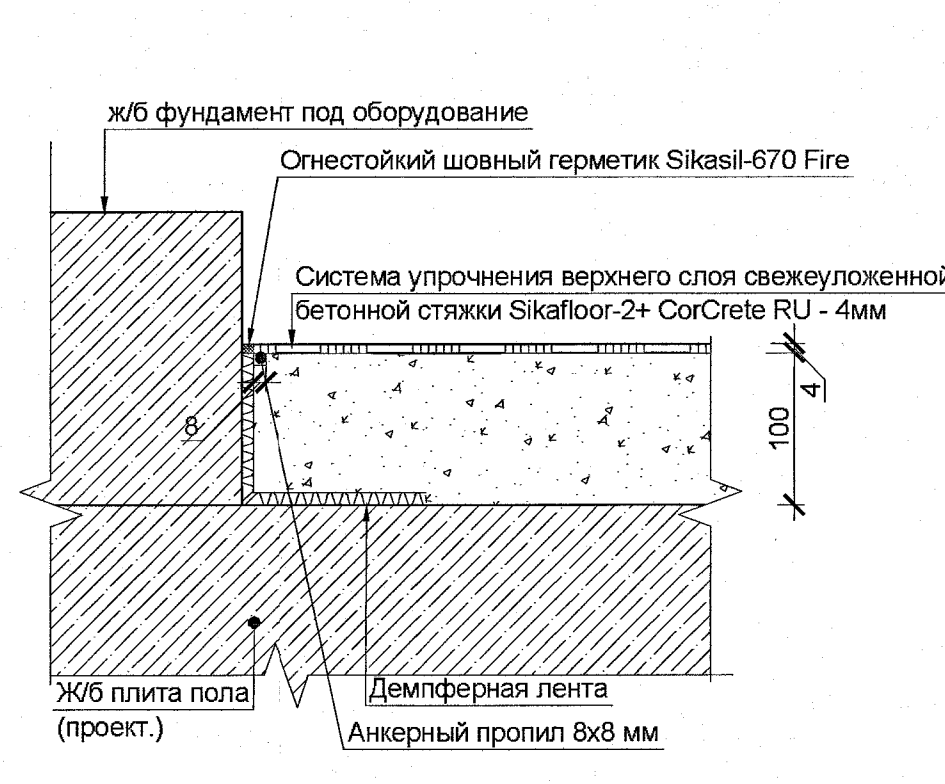
Узел примыкания покрытия пола по системе Sika к фундаменту под оборудование (для полов типа 5) М 1:10
