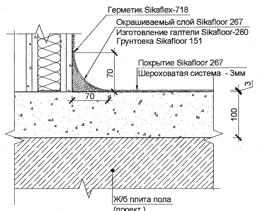
Узел примыкания покрытия пола по системе Sika к каркасной перегородке (для полов типа 6) М 1:10
