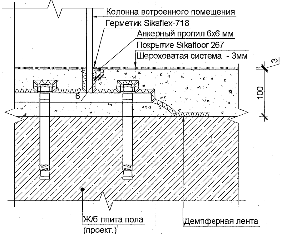
Узел примыкания покрытия пола по системе Sika к проектируемым колоннам (для полов типа 6) М 1:10
