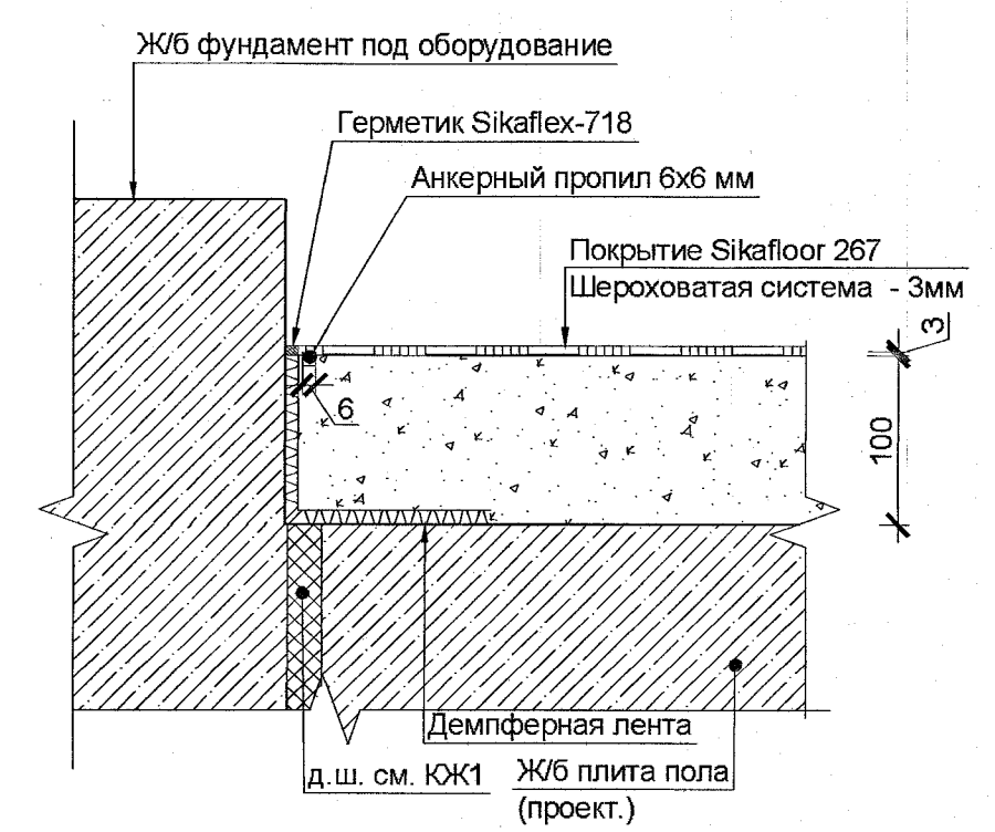
Узел примыкания покрытия пола по системе Sika к фундаменту под оборудование (для полов типа 6) М 1:10
