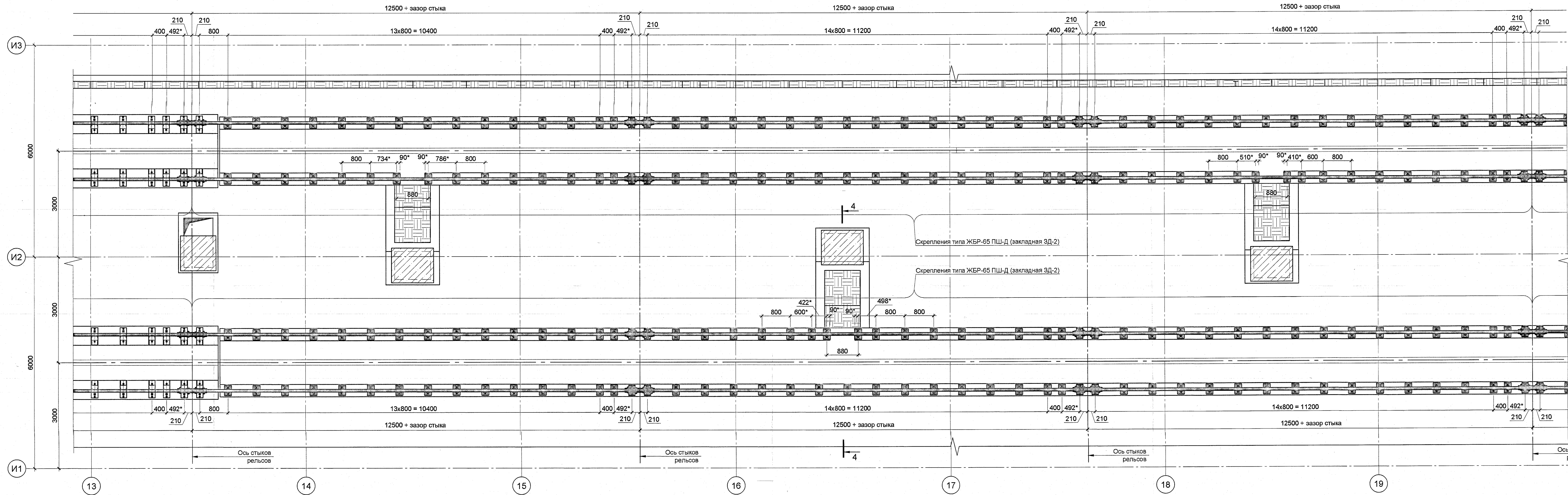
Схема расположения элементов рельсовых креплений и закладных деталей под них между осями 13-19 / И1-И3
