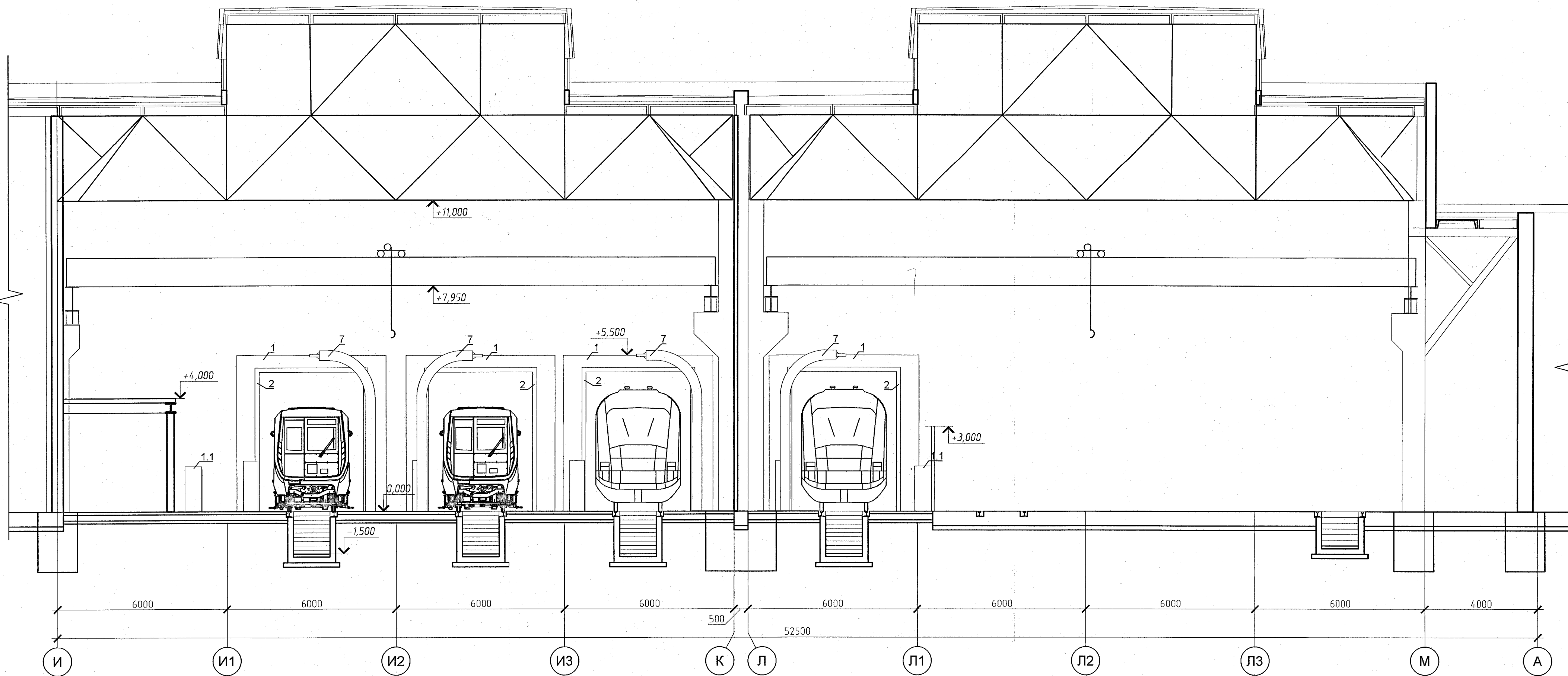
Разрез 1 - 1
