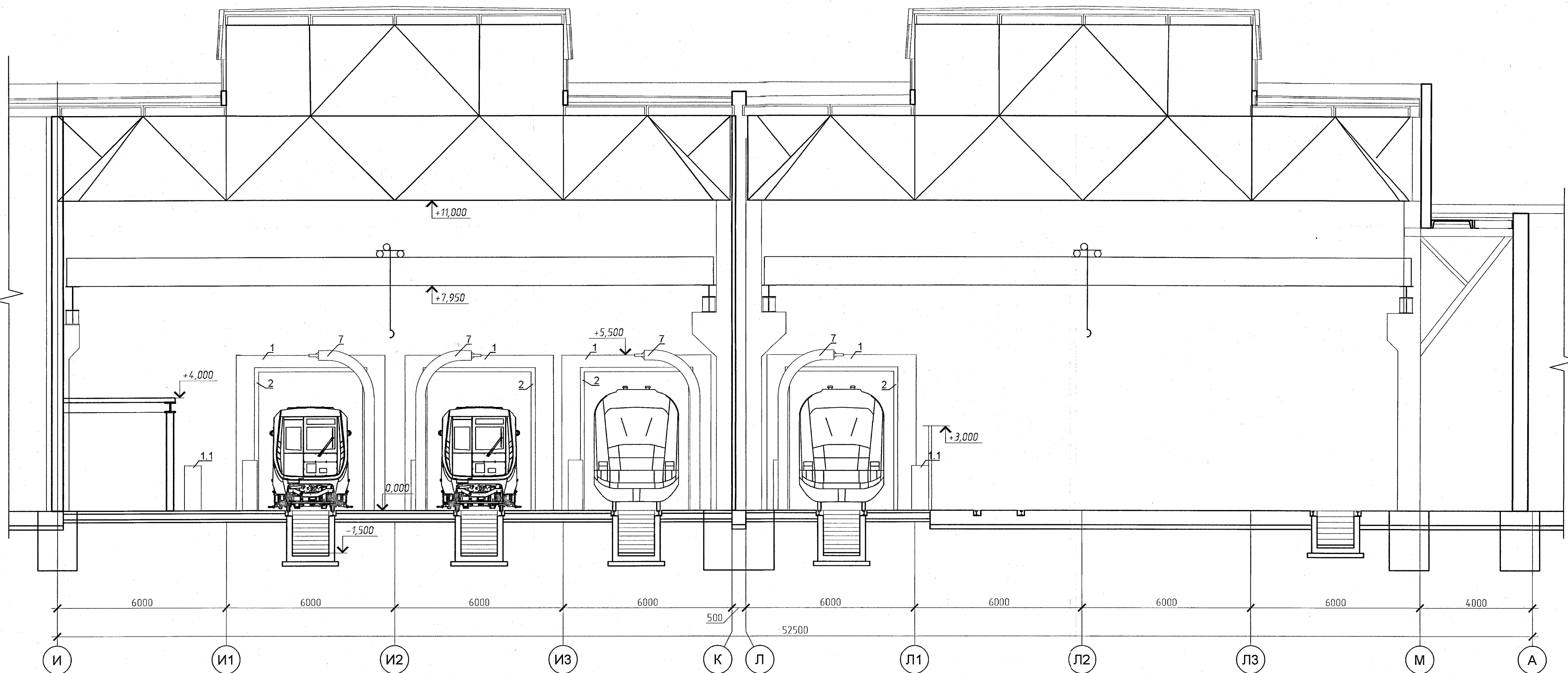
Разрез 1 - 1
