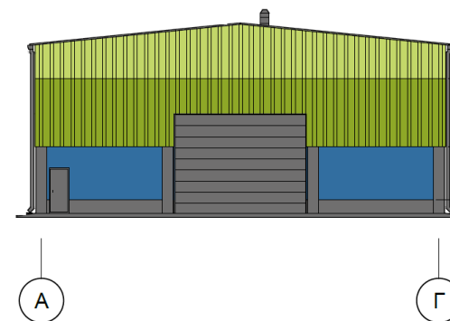
Фасад А-Г
