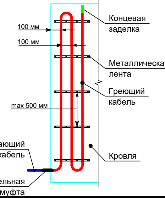
Укладка и крепление греющего кабеля
