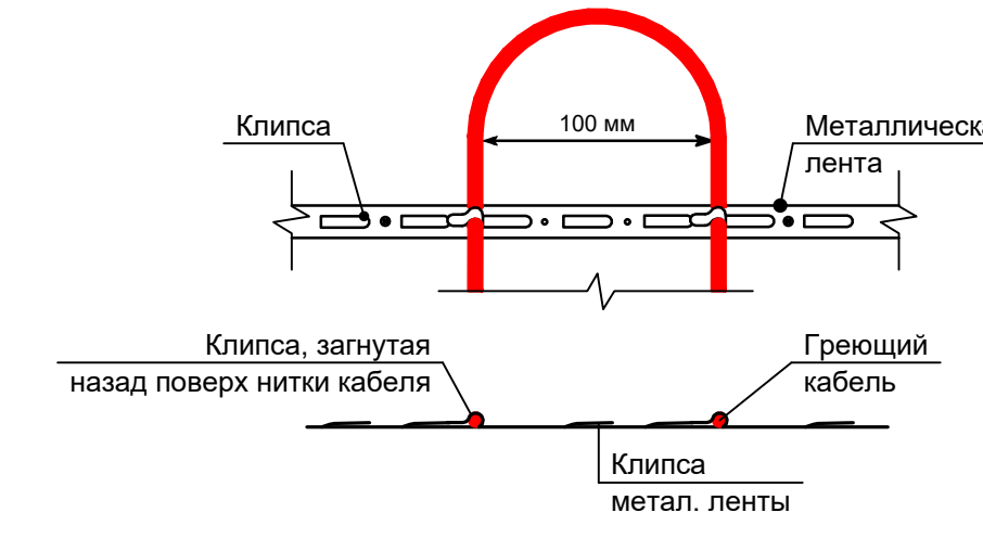
Крепление греющего кабеля
