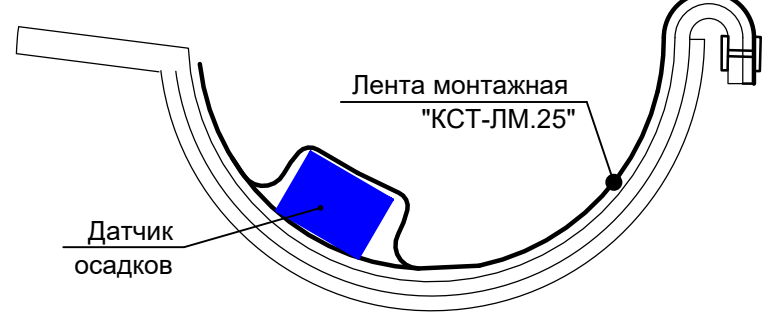
Типовой узел крепления датчика осадков в подвесных лотках
