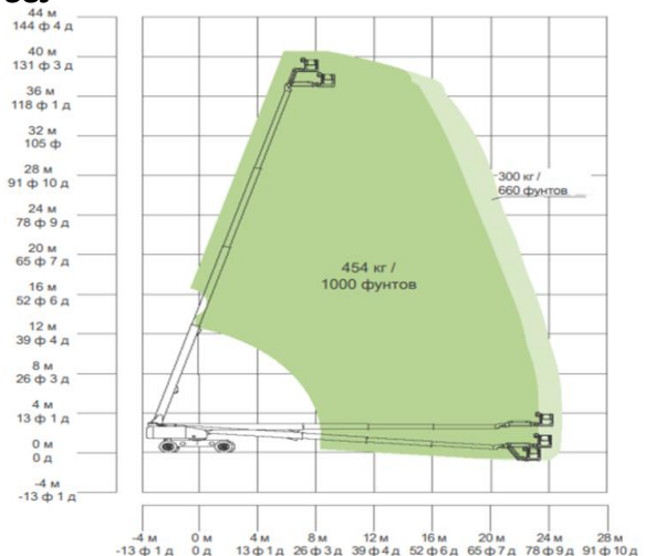
Диаграмма грузоподъемности модели Zoomlion ZT38J
