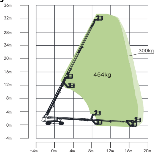
Диаграмма грузоподъемности модели Zoomlion ZT32J
