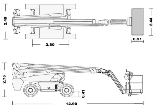
Размеры модели Zoomlion ZT32J
