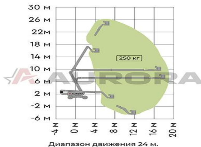
Диаграмма грузоподъемности модели Aurora ZA24J
