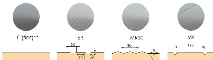
Виды профилирования поверхностей стеновых и кровельных МВ панелей:
