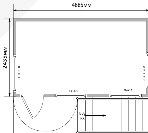
2этаж
