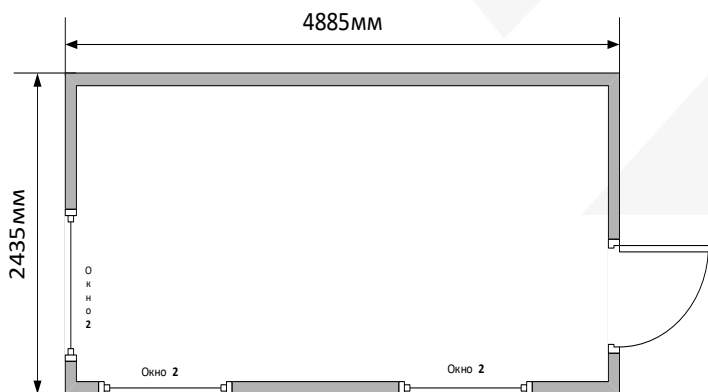
1этаж
