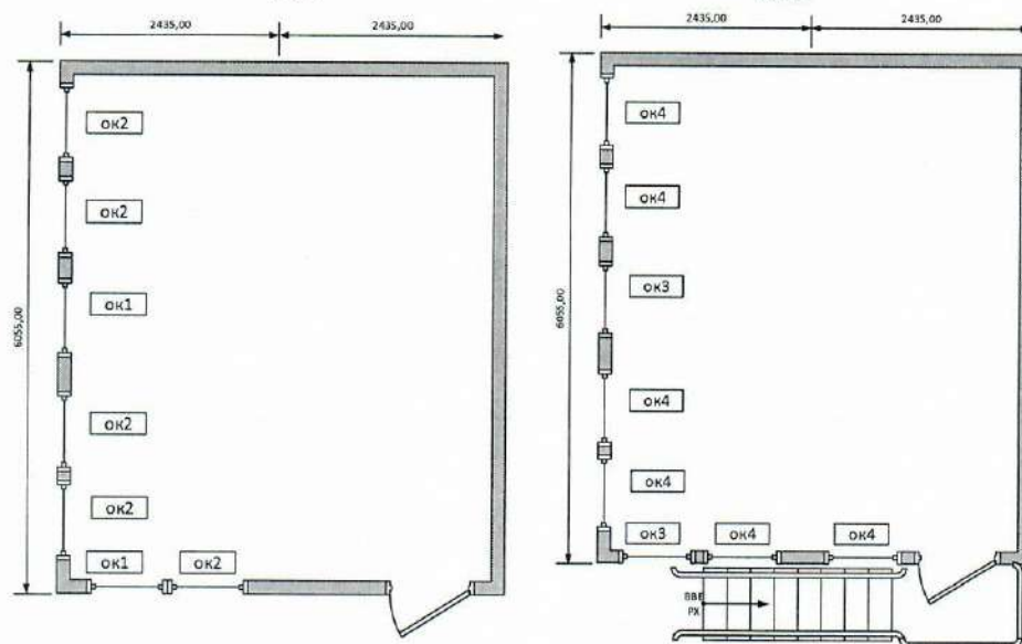
Схема планировки модульного здания
