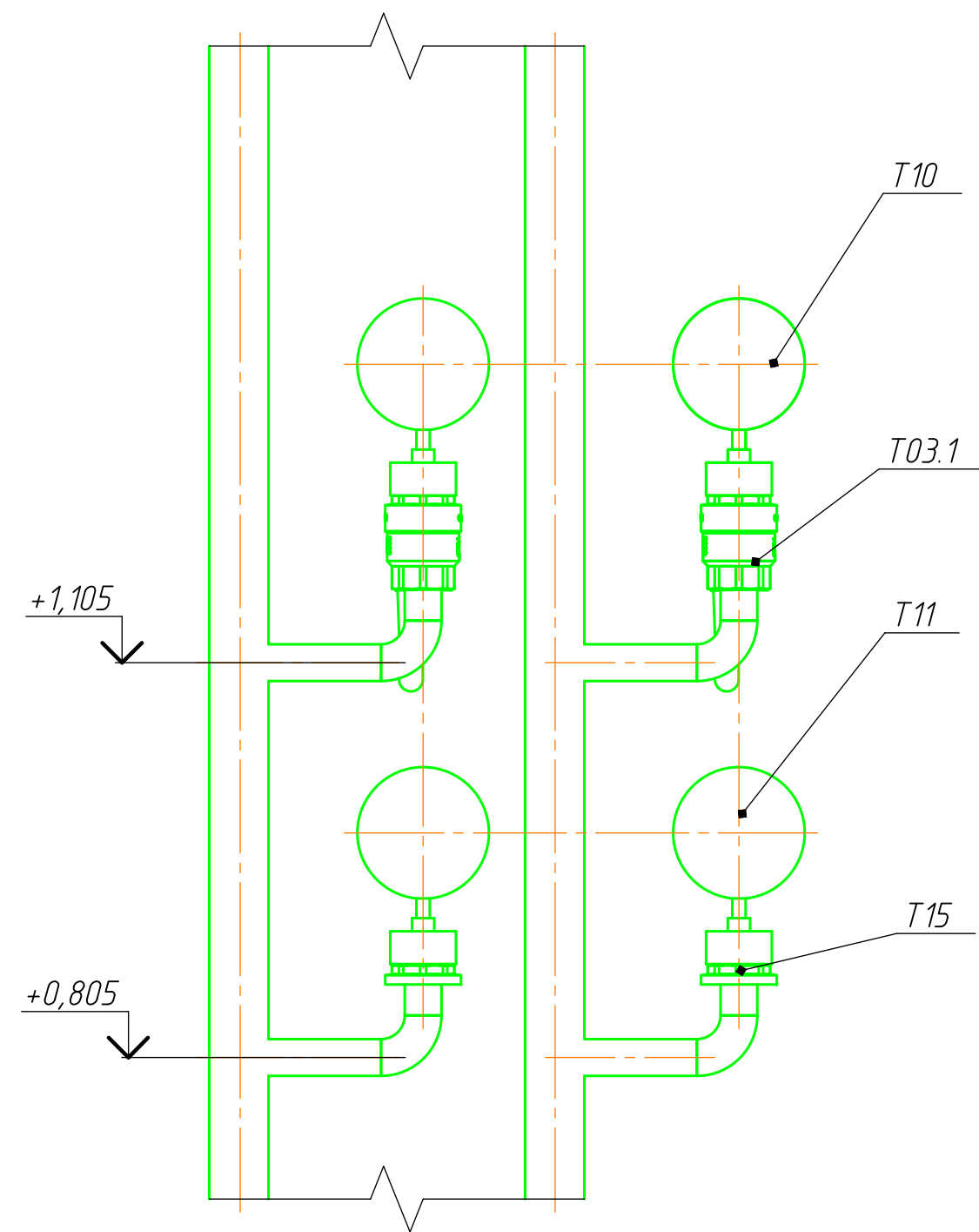
Узлы манометров и термометров T1/T2
