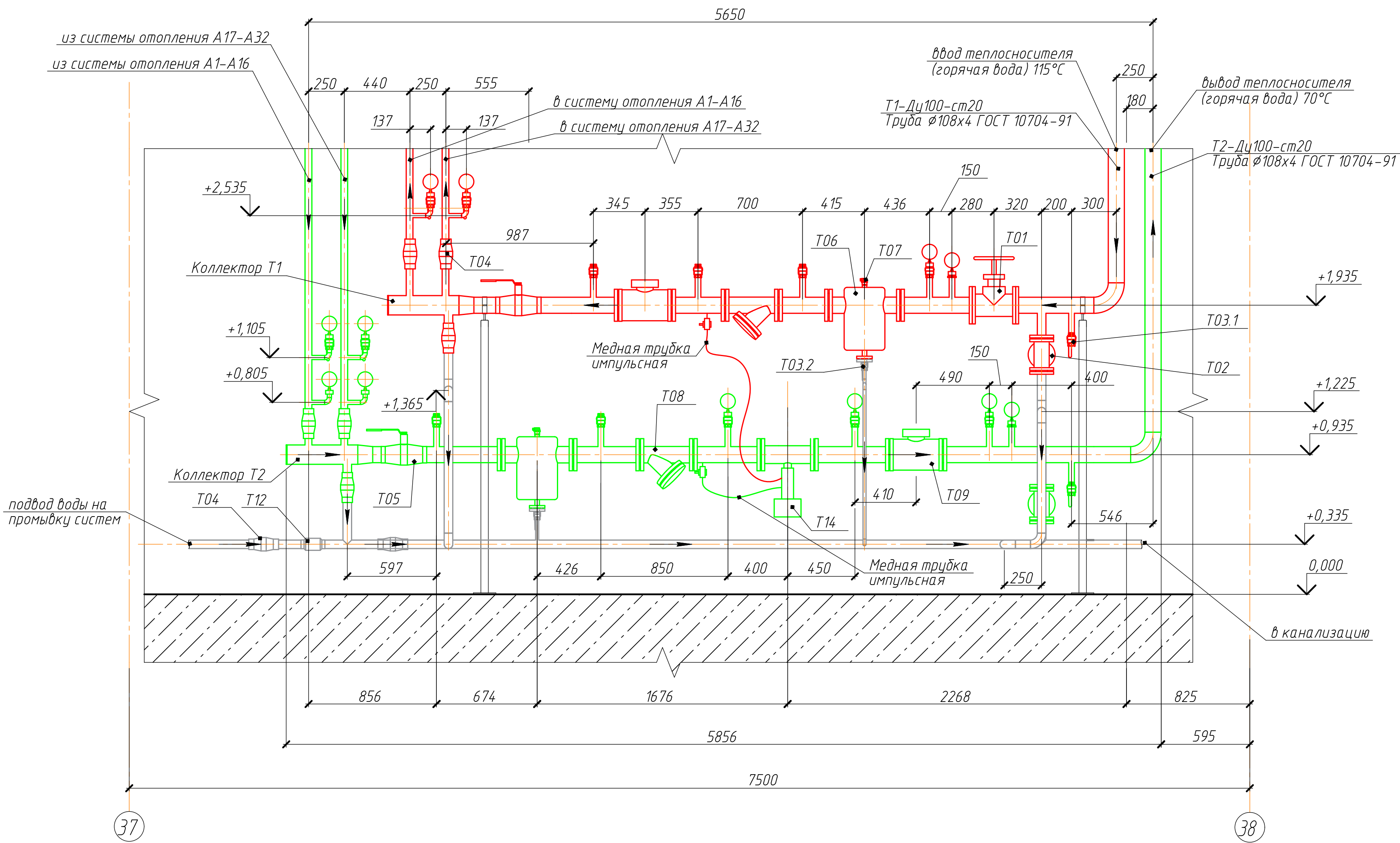
Узел управления T1/T2
