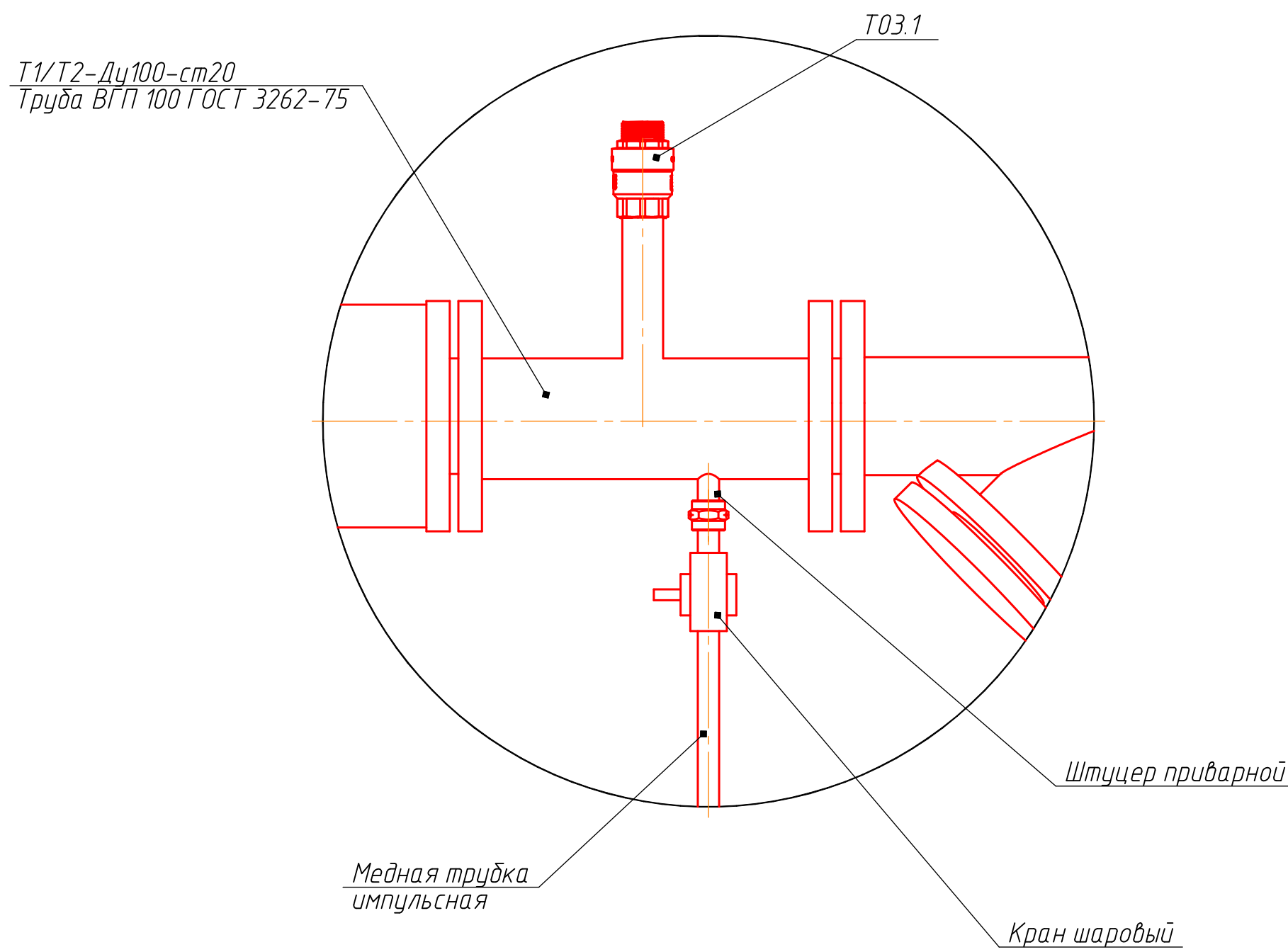
Подключение импульсных трубок к T1/T2
