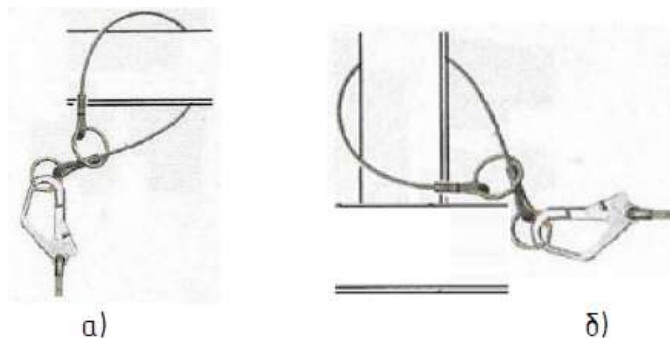
Рисунок 15.2.7. Крепление анкерного стропа: за горизонтальную металлоконструкцию (а), за вертикальную металлоконструкцию (б).
