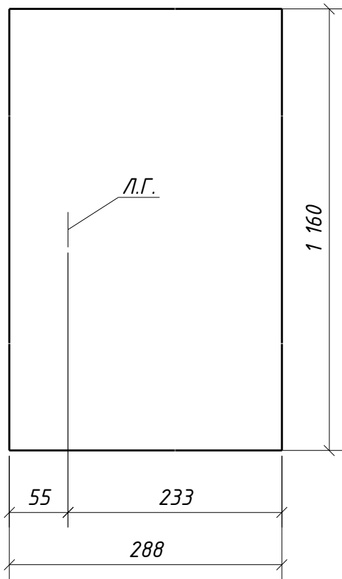
Развертка дет. 628
