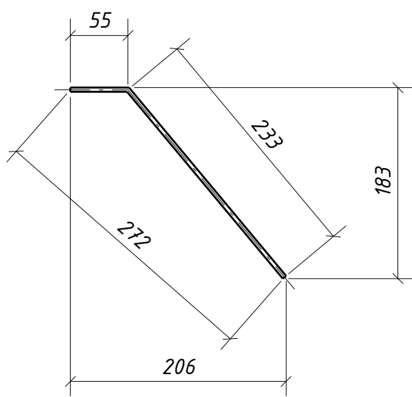
Гиб дет. 628
