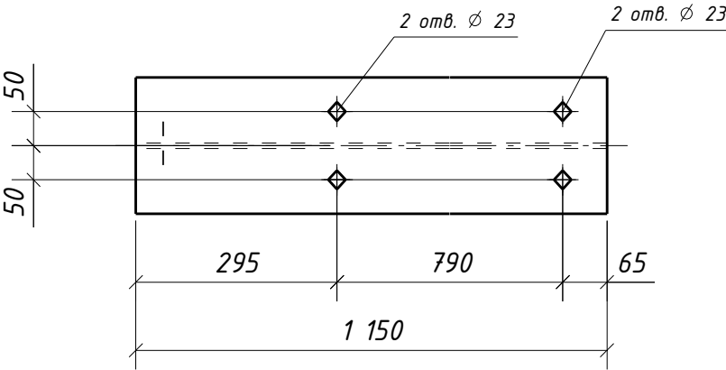
Дет. 1093
