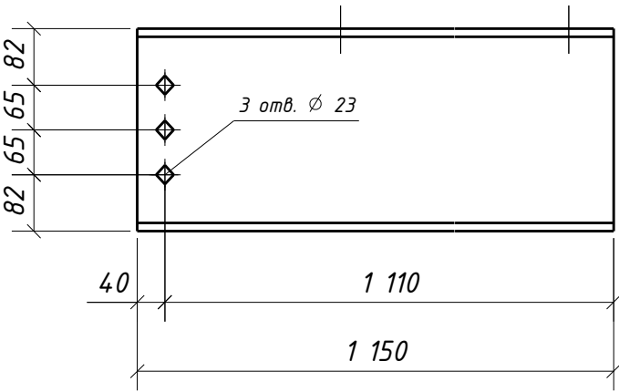
Дет. 1093
