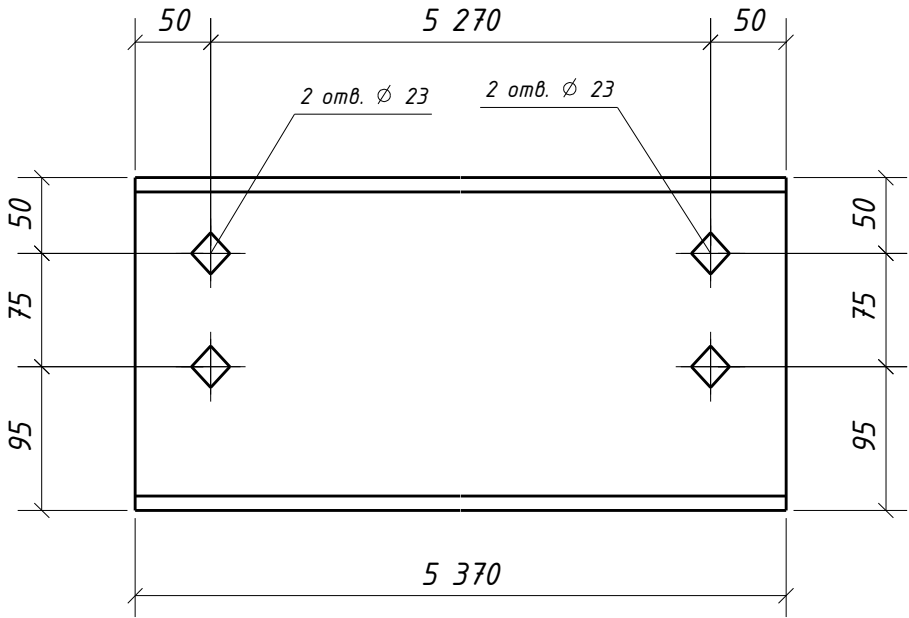
Дет. 1153
