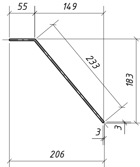
Гиб дет. 1250
